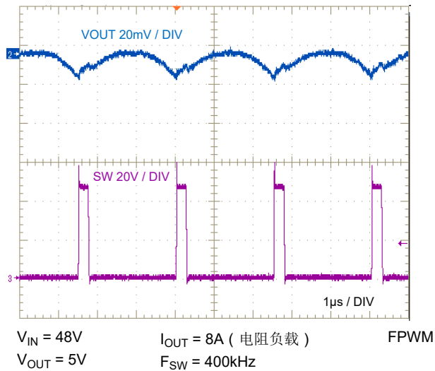
图 7-15. 满负载开关
