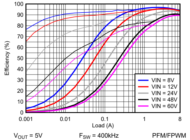
图 7-14. 效率与 I_{OUT} 间的关系，对数标度
