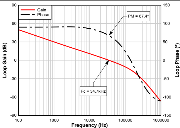
F_c = 交叉频率, PM = 相位裕度。 V_{IN} = 24V F_{SW} = 400kHz FPWM V_{OUT} = 3.3V I_{OUT} = 10A (电阻负载) L = 2.2 \mu H
