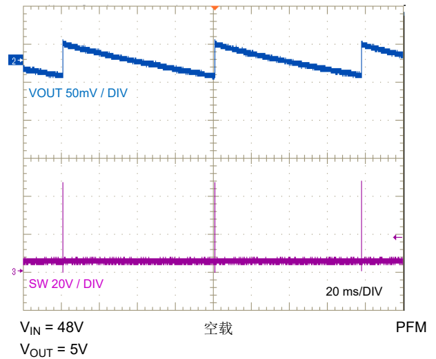
图 7-16. PFM 开关
