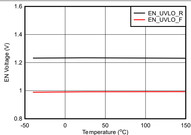
图 6-3. 启用 UVLO
