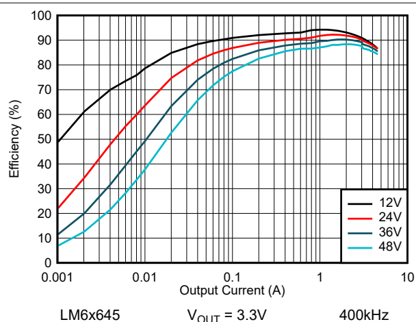
图 8-16. LM6x645 效率 — 自动模式
