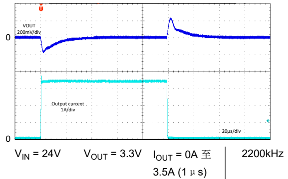
图 8-84. 负载瞬态 — LM6x635 — FPWM
