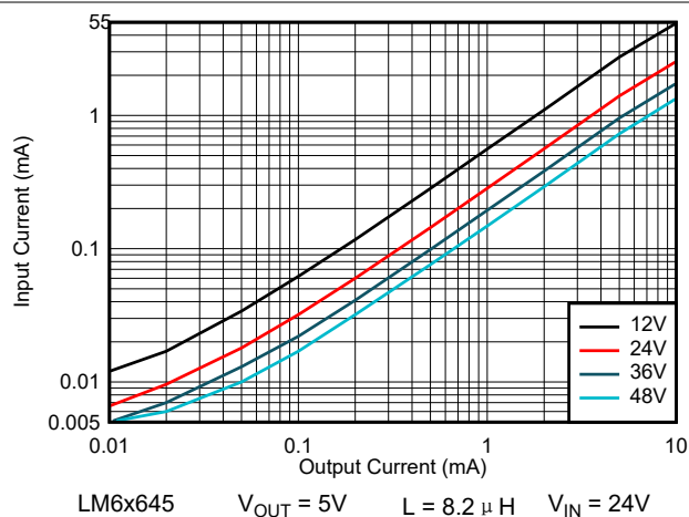
图 8-71. 输入电源电流 — 自动模式
