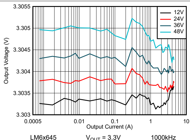
图 8-52. LM6x645 线路和负载调整 — FPWM 模式
