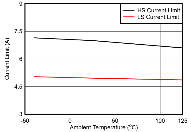
图 6-8. 4.5A 电流限制
