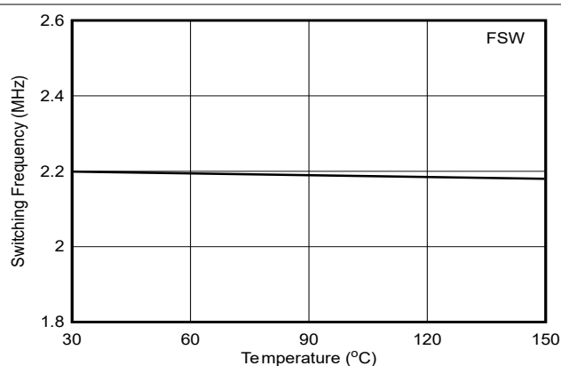
图 6-5. f_{SW} 2.2MHz
