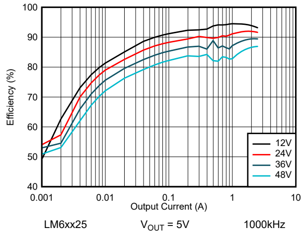
图 8-33. LM6xx25 效率 — 自动模式
