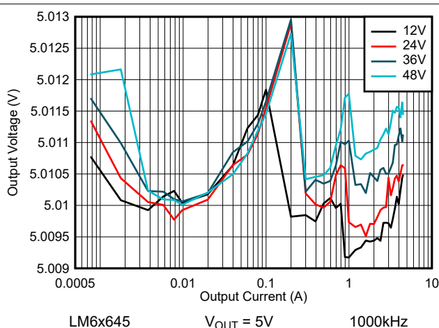
图 8-53. LM6x645 线路和负载调整 — 自动模式
