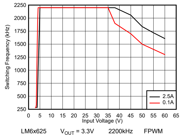
图 8-58. LM6x625 开关频率与输入电压间的关系
