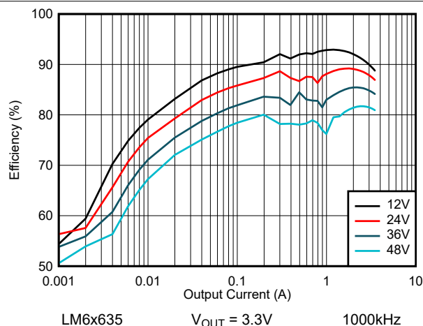
图 8-35. LM6x635 效率 — 自动模式
