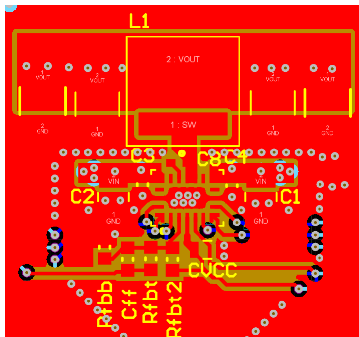
图 8-98. 布局示例
