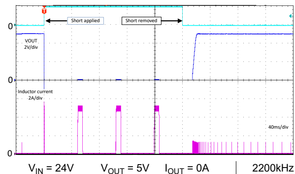
图 8-89. 输出短路电流和恢复 — 自动
