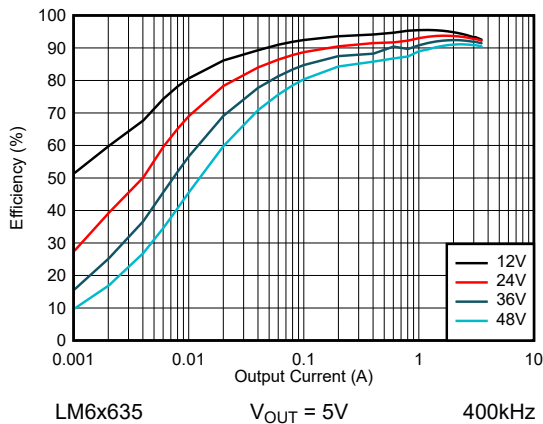
图 8-11. LM6x635 效率 — 自动模式
