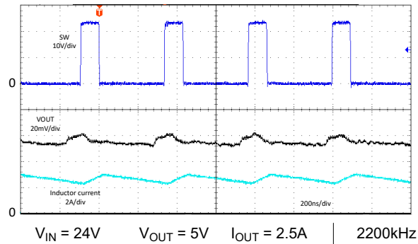
图 8-81. 典型开关波形 — LM6x625 — FPWM
