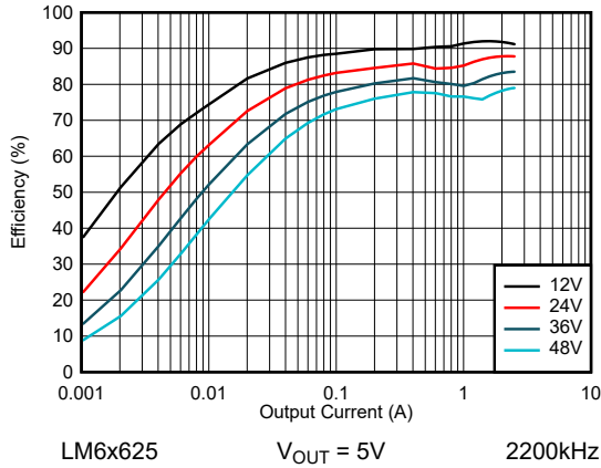
图 8-9. LM6x625 效率 — 自动模式
