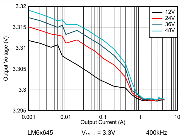
图 8-28. LM6x645 线路和负载调整 — 自动模式
