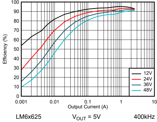
图 8-7. LM6x625 效率 — 自动模式
