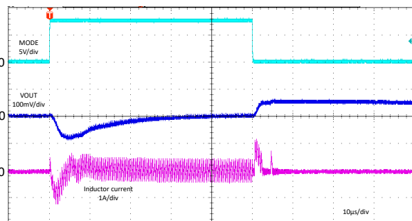
图 8-91. 模式变化瞬态
