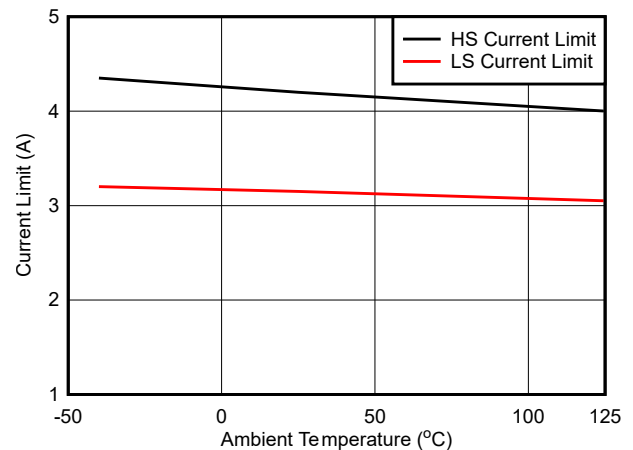
图 6-10. 2.5A 电流限制
