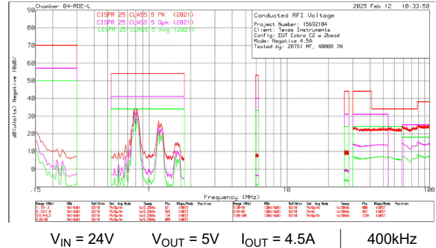
图 8-80. LM6x645 传导 EMI — 负线路
