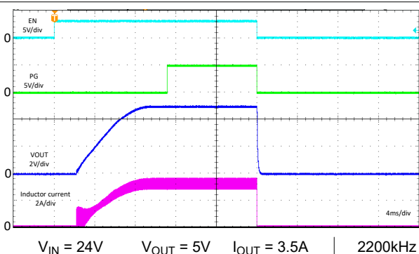
图 8-88. 启动/关断 — FPWM
