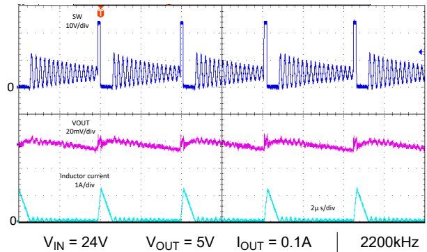
图 8-82. 典型开关波形 — LM6x625 — 自动
