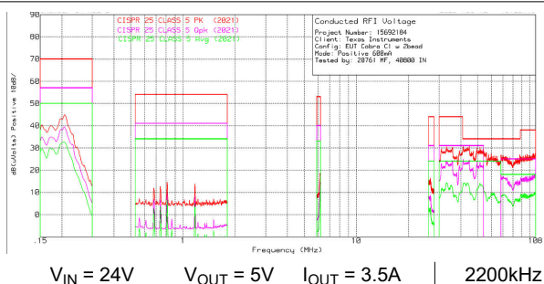
图 8-77. LM6x635 传导 EMI — 正线路
