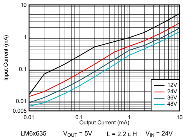
图 8-69. 输入电源电流 — 自动模式
