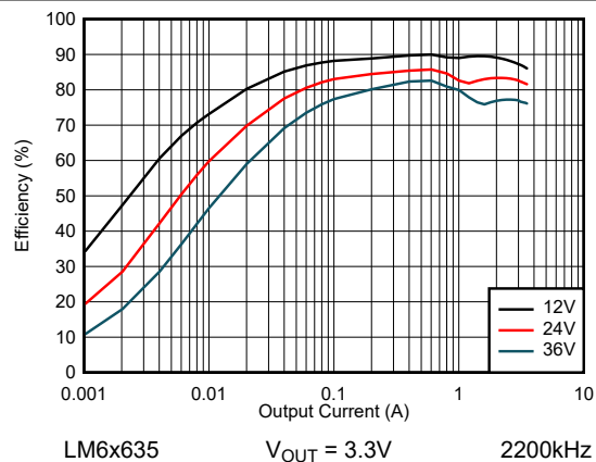
图 8-14. LM6x635 效率 — 自动模式
