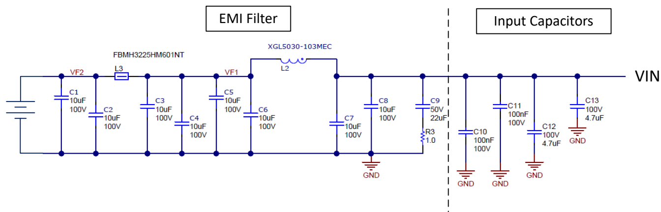
图 8-96. 400kHz 的 EMI 输入滤波器
