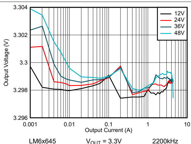
图 8-30. LM6x645 线路和负载调整 — 自动模式
