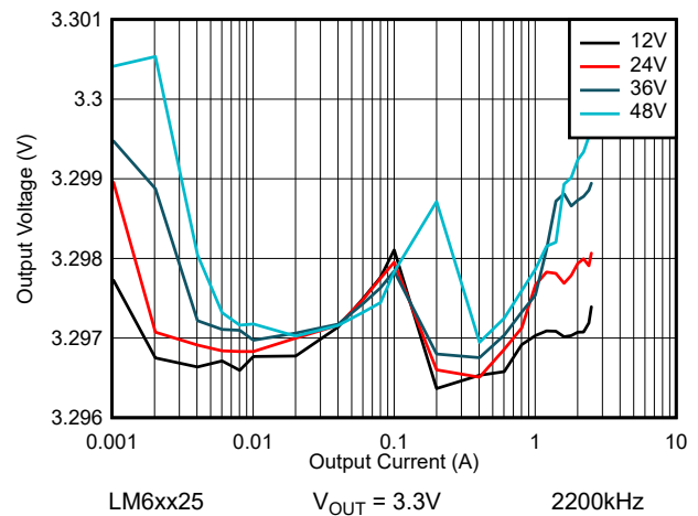
图 8-22. LM6xx25 线路和负载调整 — 自动模式
