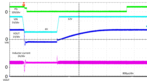
图 8-92. 压降瞬态和恢复
