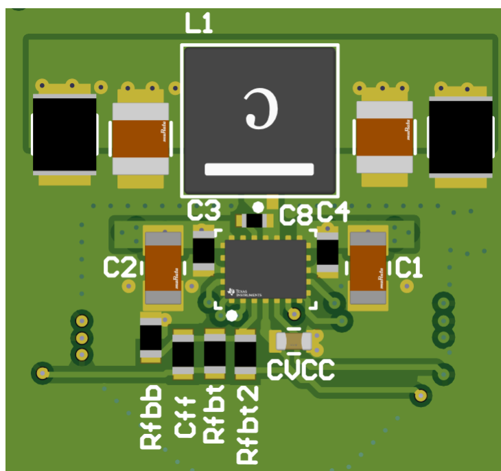
图 8-99. PCB 图像
