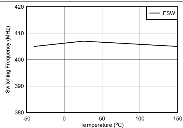
图 6-6. f_{SW} 400kHz
