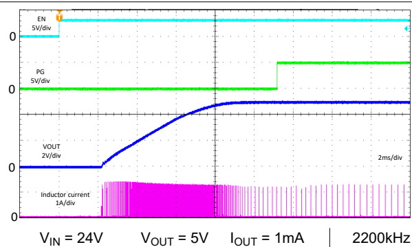
图 8-87. 启动 — 自动
