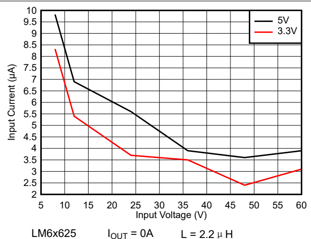
图 8-72. 空载输入电源电流 — 自动模式
