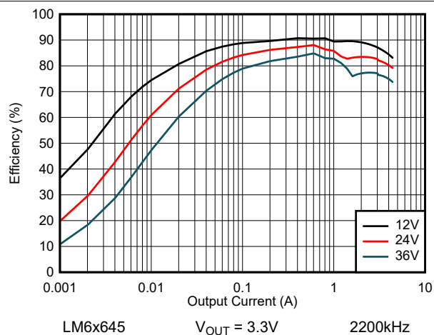
图 8-18. LM6x645 效率 — 自动模式
