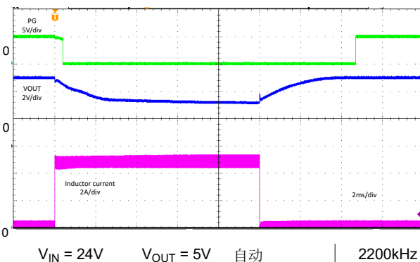
图 8-90. 电流限值瞬态
