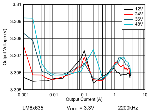
图 8-26. LM6x635 线路和负载调整 — 自动模式
