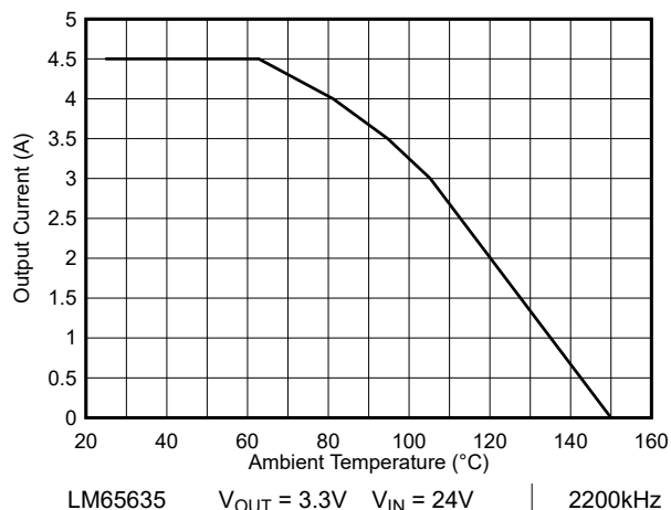
图 8-6. 热降额 — 2200kHz
