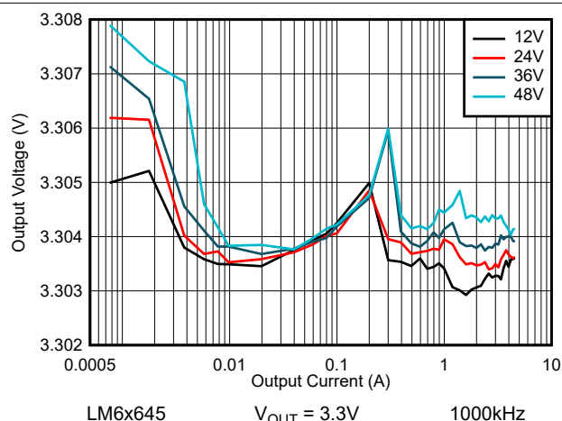
图 8-51. LM6x645 线路和负载调整 — 自动模式
