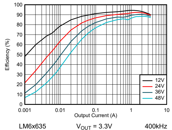
图 8-12. LM6x635 效率 — 自动模式
