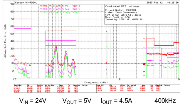
图 8-79. LM6x645 传导 EMI — 正线路
