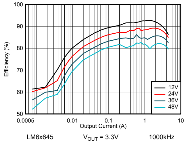
图 8-39. LM6x645 效率 — 自动模式
