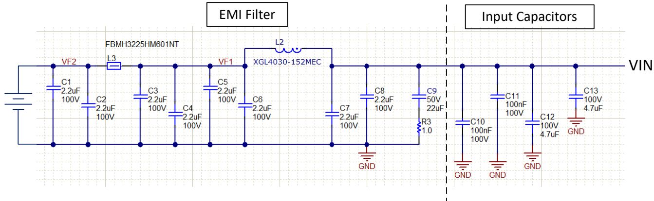
图 8-95. 2200kHz 的 EMI 输入滤波器
