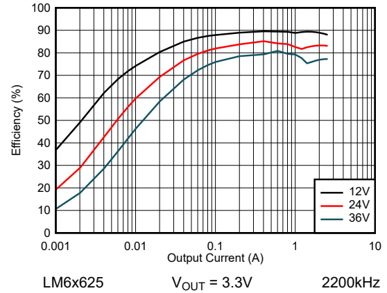
图 8-10. LM6x625 效率 — 自动模式
