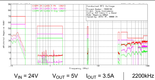
图 8-78. LM6x635 传导 EMI — 负线路
