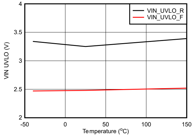
图 6-7. V_{IN} UVLO
