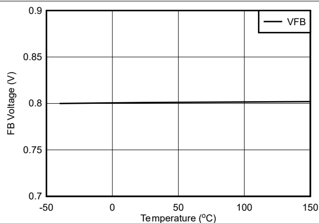
图 6-1. 反馈电压
