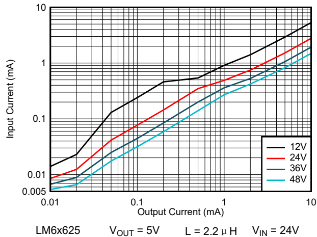
图 8-67. 输入电源电流 — 自动模式
