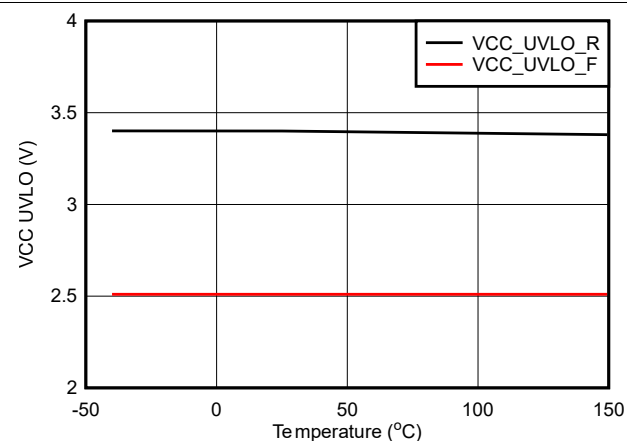
图 6-4. V_{CC} UVLO
