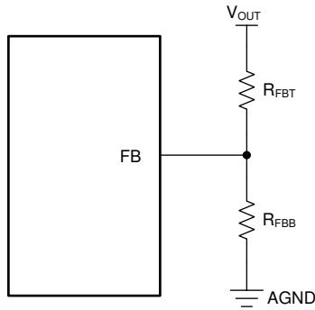
图 7-3. 设置可调版本的输出电压
