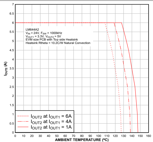
图 8-6. 典型输出电流与环境温度间的关系，VIN = 24V，FSW = 1MHz，双路输出
