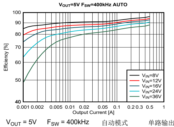
图 8-9. 效率
