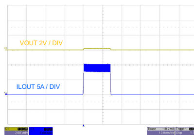
图 8-42. 短路保护
