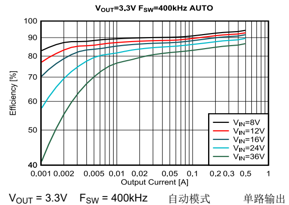
图 8-12. 效率
