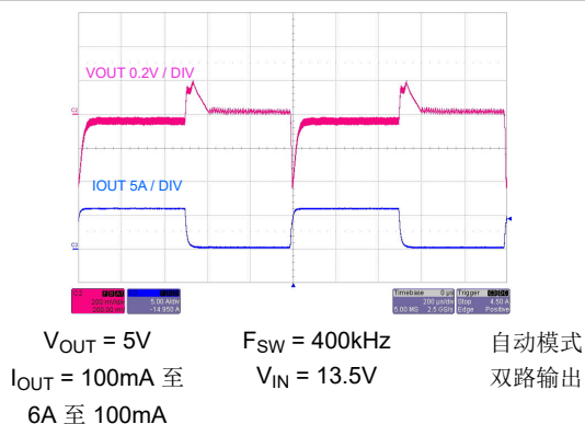
图 8-47. 负载瞬态
