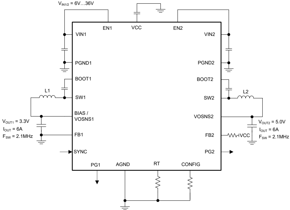
图 7-1. 输入电压工作范围为 6V 至 36V 时的双路输出稳压器原理图
