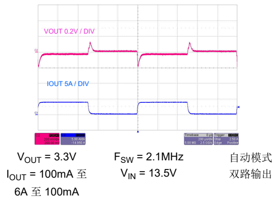
图 8-50. 负载瞬态
