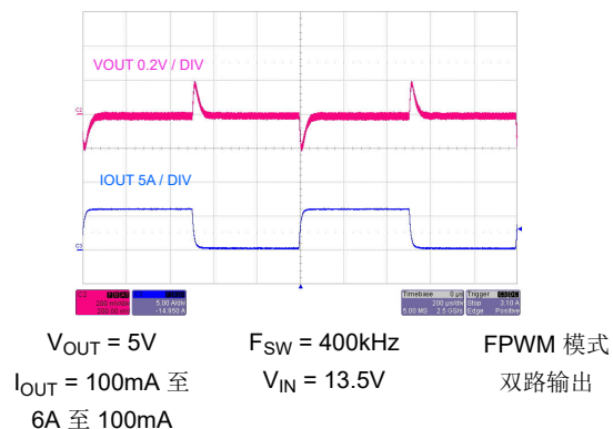
图 8-46. 负载瞬态
