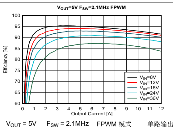
图 8-17. 效率
