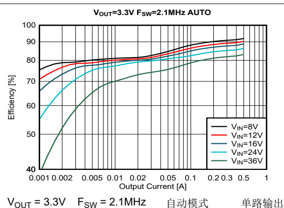
图 8-18. 效率
