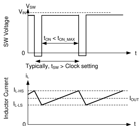
图 7-15. 电流限值波形
