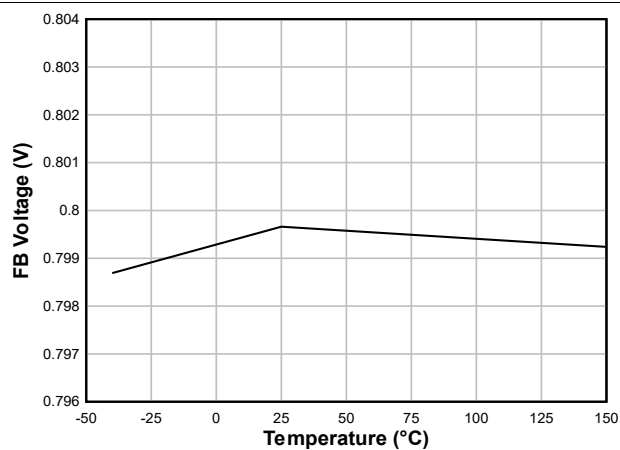
图 6-1. 反馈电压
