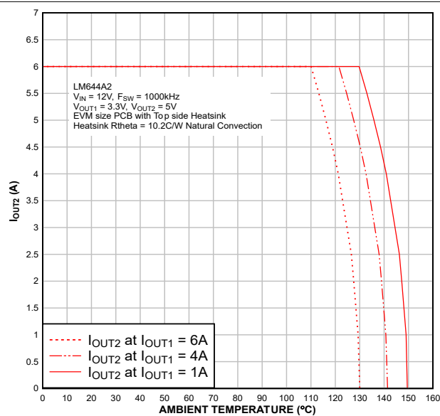
图 8-5. 典型输出电流与环境温度间的关系，VIN = 12V，FSW = 1MHz，双路输出
