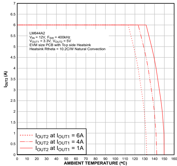
图 8-3. 典型输出电流与环境温度间的关系，VIN = 12V，FSW = 400kHz，双路输出
