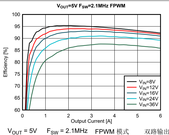
图 8-23. 效率
