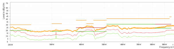
图 8-57. 单输出单极辐射发射与 CISPR25 5 类限值间的关系 ( 橙色：峰值信号，红色：平均信号，绿色：准峰值信号 )
