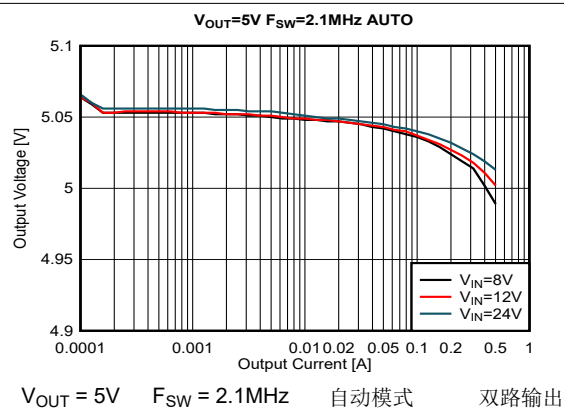
图 8-32. 负载调整率和线性调整率
