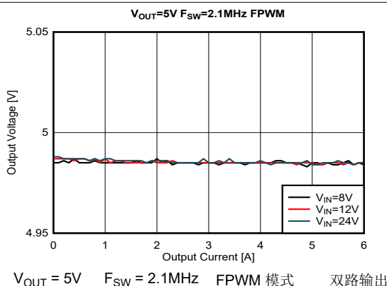
图 8-31. 负载调整率和线性调整率
