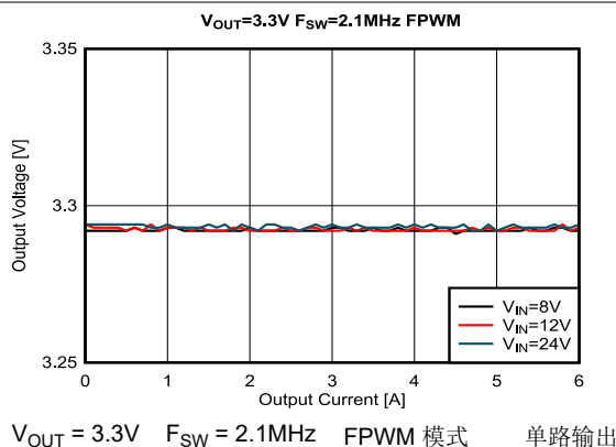
图 8-27. 负载调整率和线性调整率
