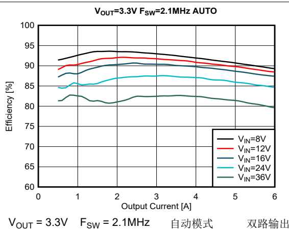
图 8-25. 效率
