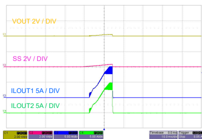
图 8-41. 短路保护
