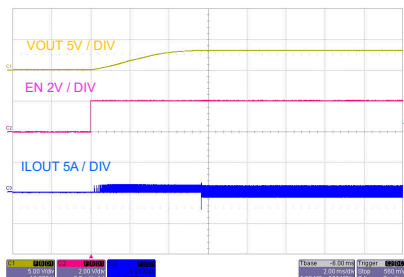
图 8-39. 在 100mA 负载下启动
