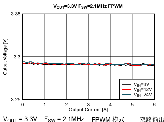
图 8-29. 负载调整率和线性调整率
