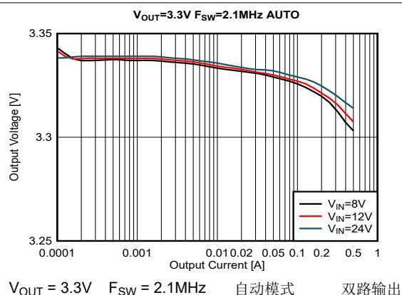
图 8-30. 负载调整率和线性调整率
