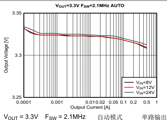
图 8-28. 负载调整率和线性调整率
