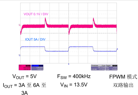
图 8-48. 负载瞬态
