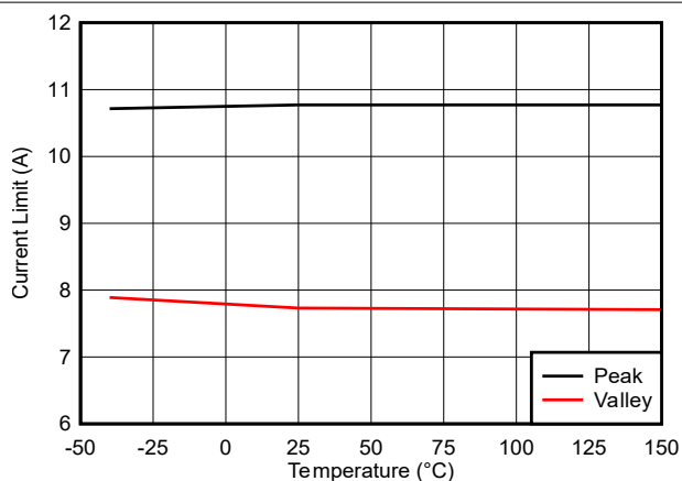
图 6-4. 高侧和低侧电流限值 LM644A2
