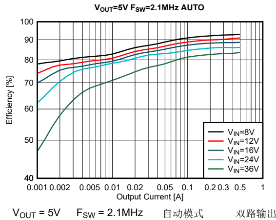
图 8-21. 效率
