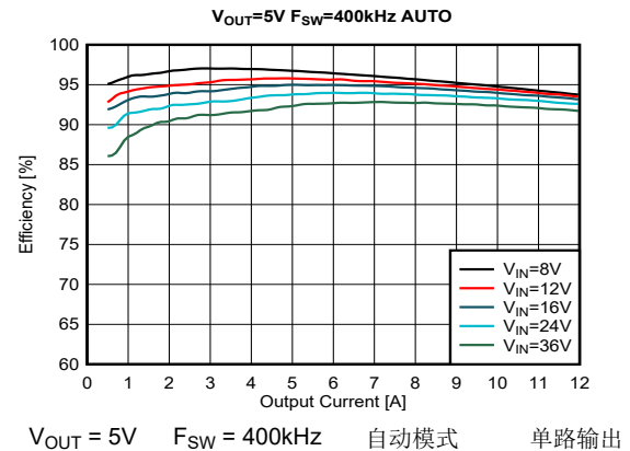
图 8-10. 效率
