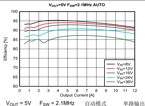
图 8-16. 效率
