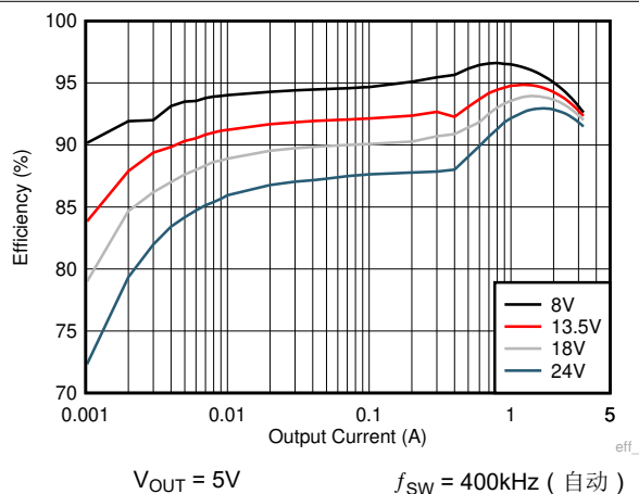
图 8-7. 效率
