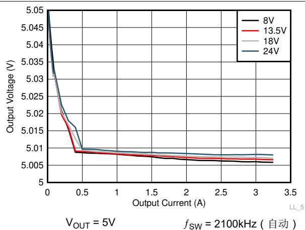
图 8-9. 线性 and 负载调整率
