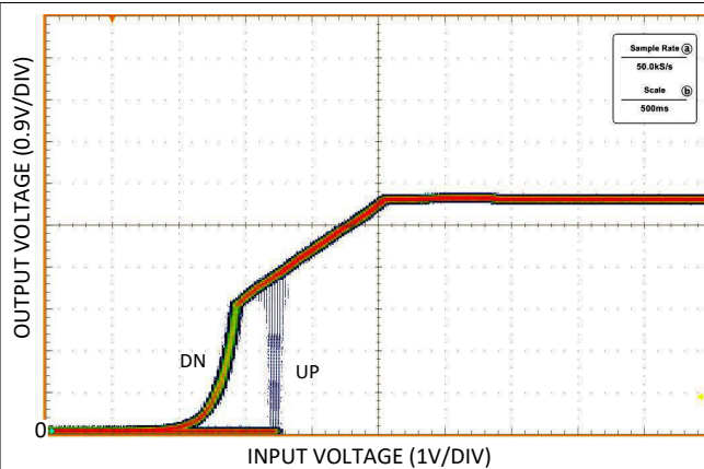
图 6-2. UVLO 阈值
