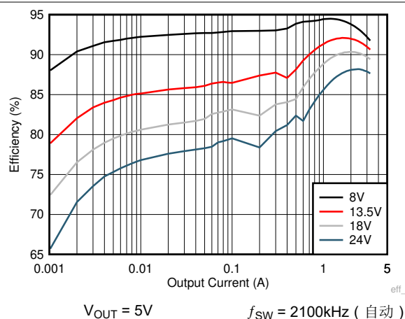
图 8-5. 效率
