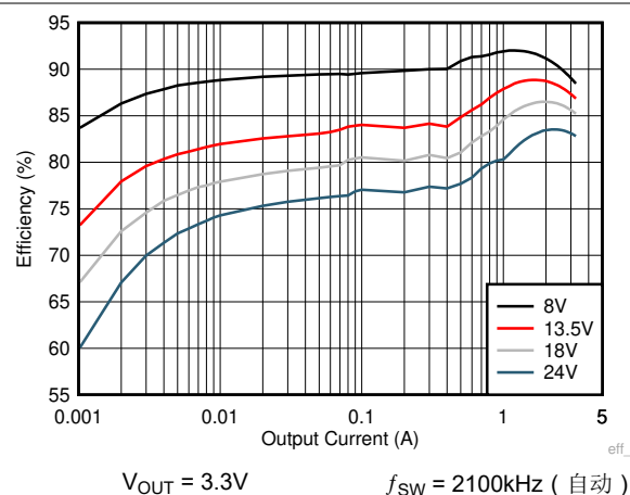
图 8-6. 效率
