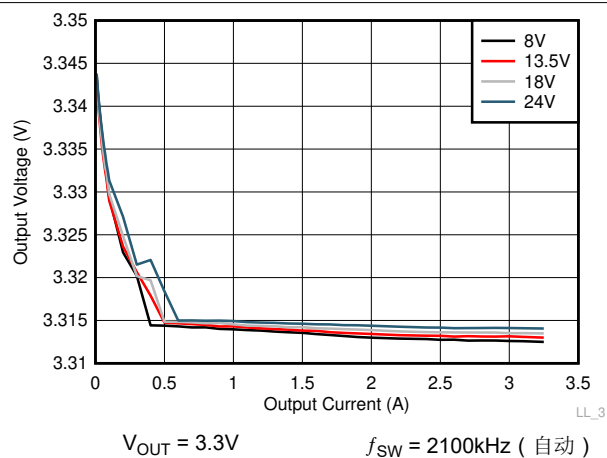
图 8-10. 线性 and 负载调整率
