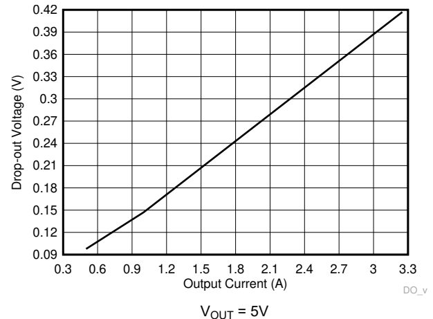
图 8-12. -1% 压降时电压降与输出电流间的关系
