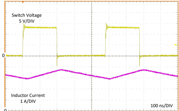
图 7-6. 没有展频的典型 PWM 开关波形， V_{IN} = 12V ， V_{OUT} = 5V ， I_{OUT} = 3.25A ， f_{SW} = 2100kHz
