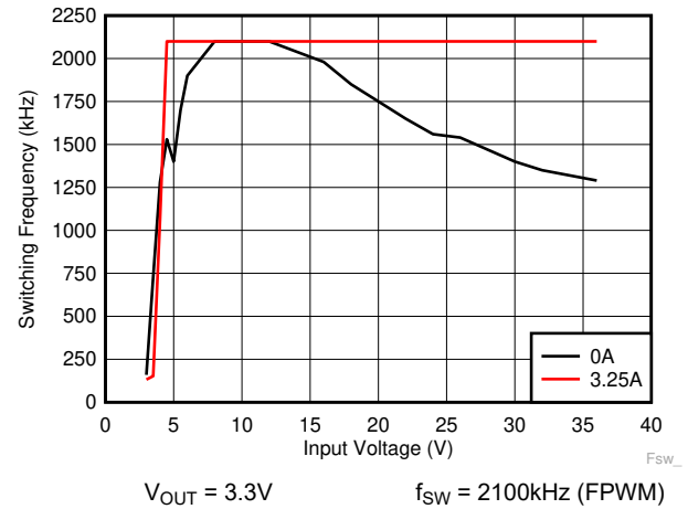
图 8-15. 开关频率与输入电压间的关系
