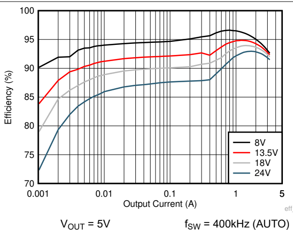
图 8-10. 效率
