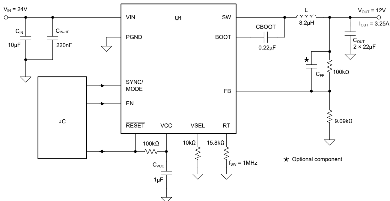
图 8-7. 全功能设计示例 V_{IN} = 24V 、 V_{OUT} = 12V 、 I_{OUT} = 3.25A 、 f_{sw} = 1MHz
