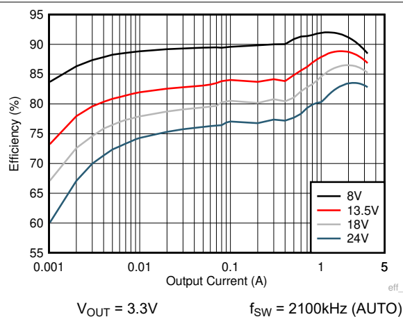
图 8-9. 效率
