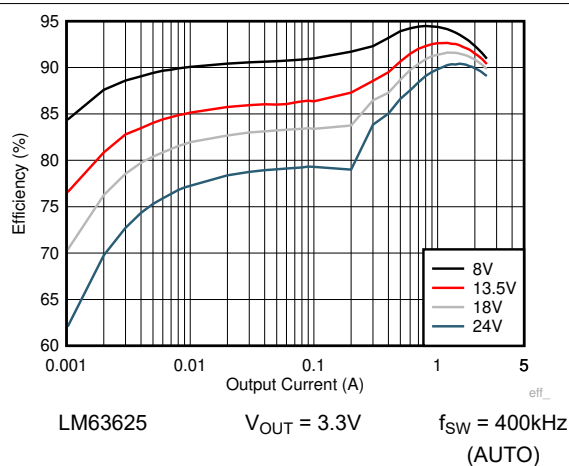
图 8-12. 效率
