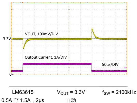
图 8-31. 负载瞬态
