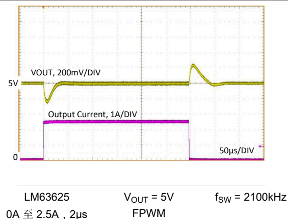
图 8-28. 负载瞬态
