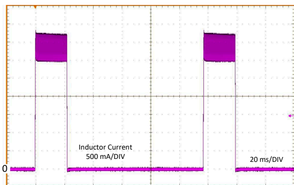
图 7-12. 短路模式下的电感器电流突发；LM63625
