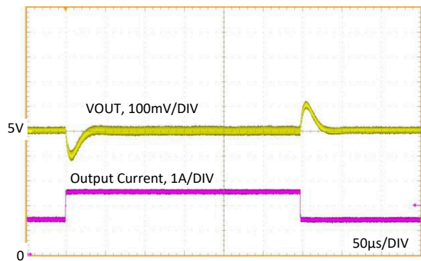
LM63625 V_{OUT} = 5V f_{SW} = 2100kHz 1.5A 至 2.5A, 2µs 自动
