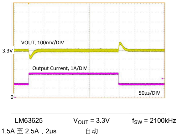
图 8-30. 负载瞬态
