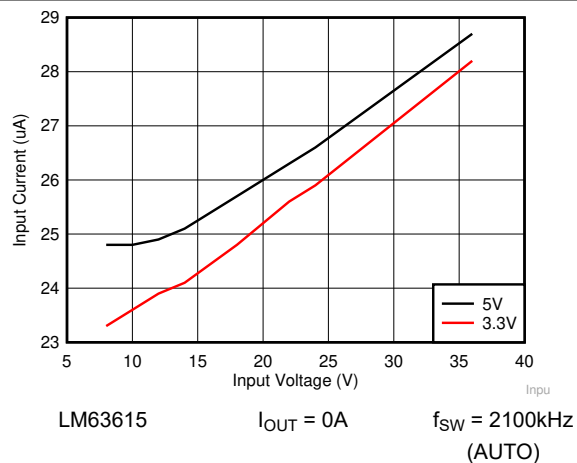
图 8-39. 输入电源电流与输入电压间的关系
