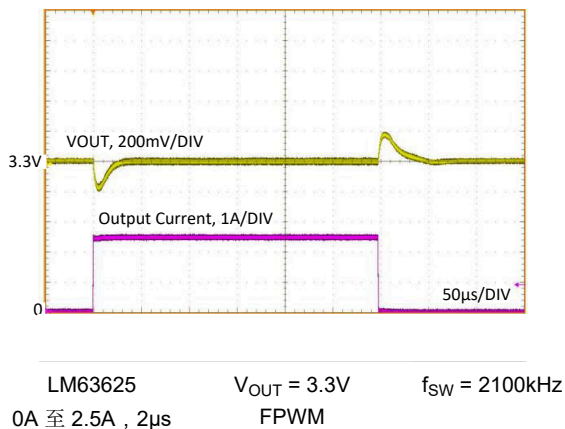
图 8-26. 负载瞬态
