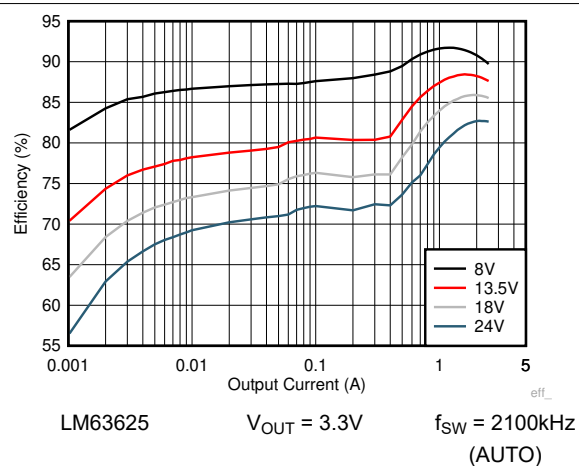
图 8-13. 效率
