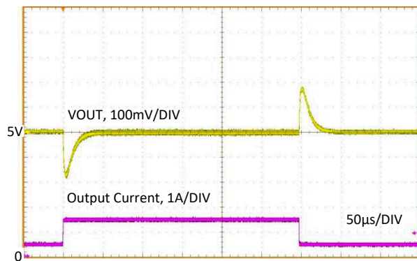
LM63615 V_{OUT} = 5V f_{SW} = 2100kHz 0.5A 至 1.5A, 2µs 自动
