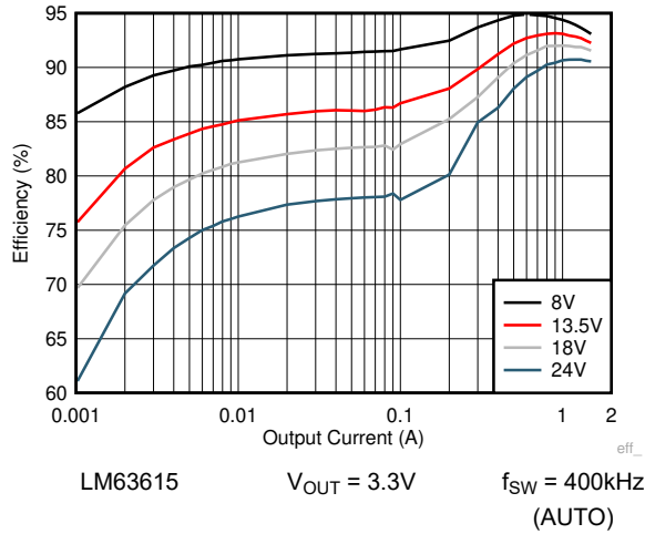
图 8-14. 效率
