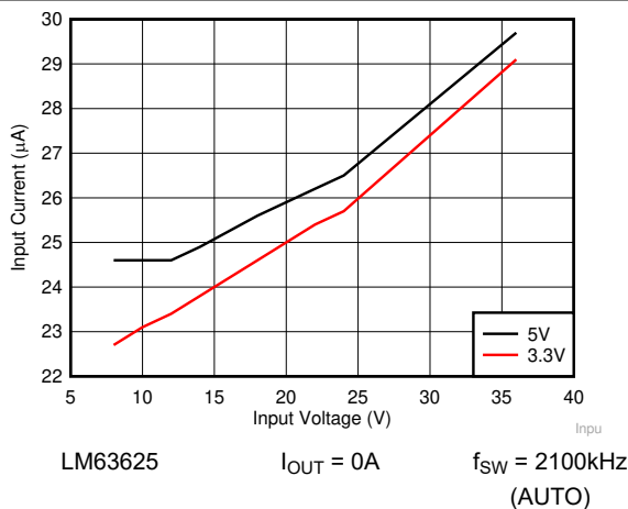
图 8-38. 输入电源电流与输入电压间的关系
