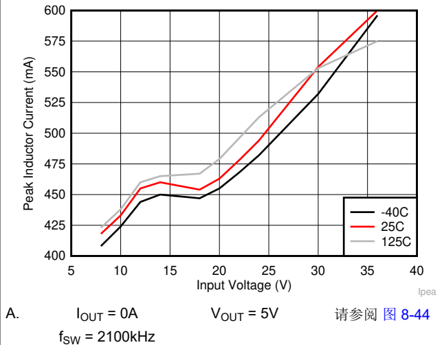
图 6-4. LM63615 的 I_{PEAK-MIN}
