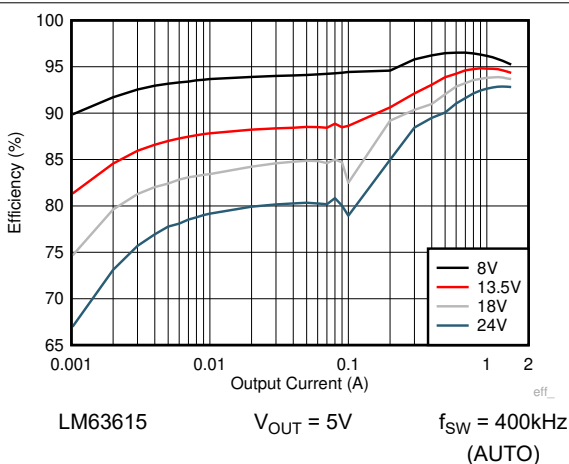
图 8-10. 效率
