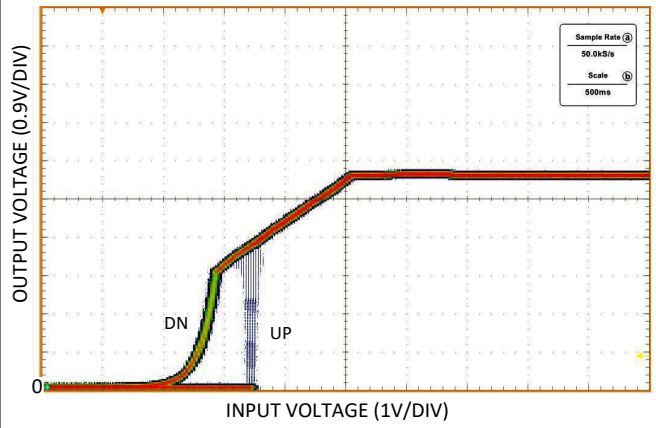
图 6-2. UVLO 阈值
