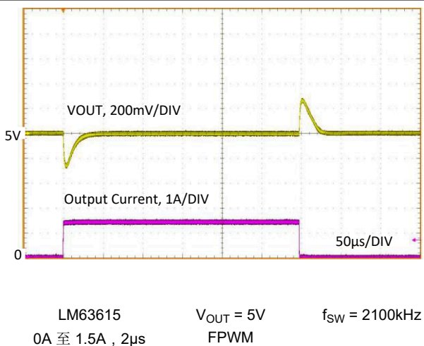
图 8-29. 负载瞬态
