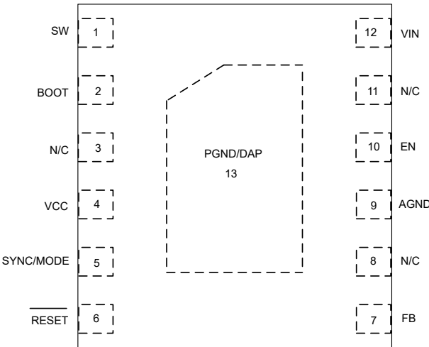
图 5-3. 具有 PowerPAD™ 集成电路封装的 12 引脚 WSON 封装 DRR — LM636x5C (顶视图)
