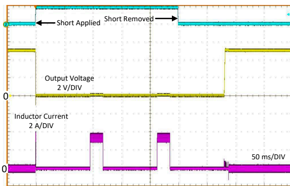
图 7-13. 短路瞬态和恢复；LM63625
