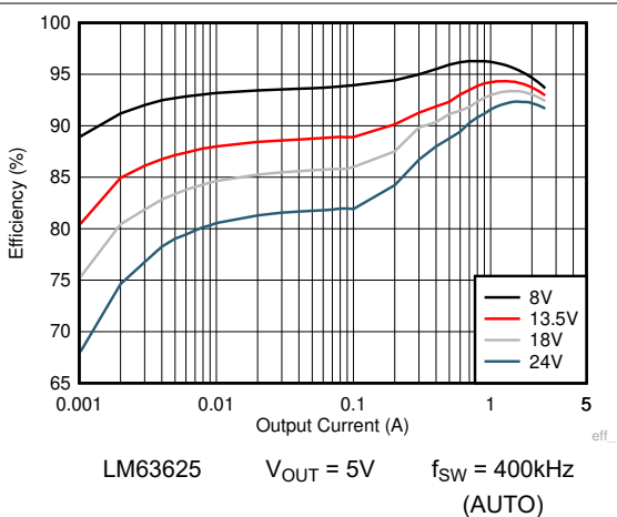
图 8-8. 效率
