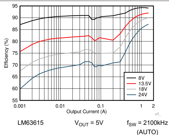
图 8-11. 效率
