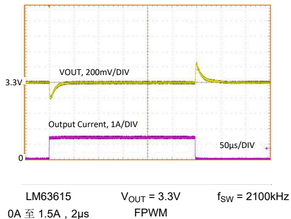
图 8-27. 负载瞬态
