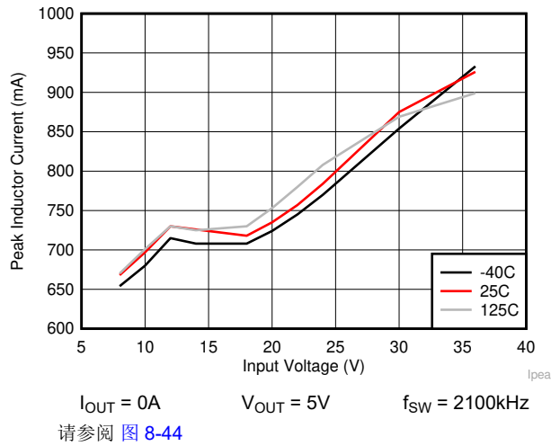
图 6-3. LM63625 的 I_{PEAK-MIN}
