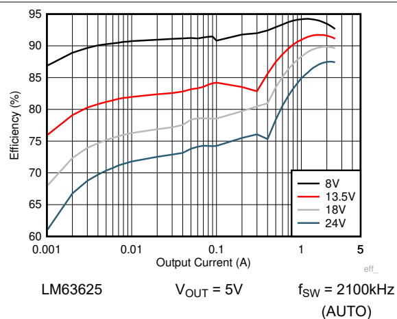
图 8-9. 效率
