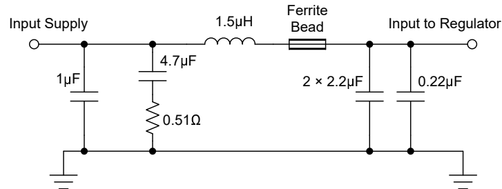
图 8-47. 典型输入 EMI 滤波器
