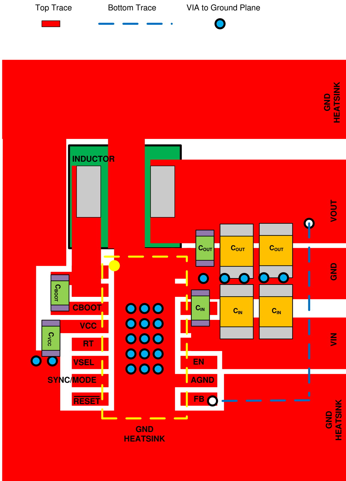
图 8-49. HTSSOP 封装的布局示例
