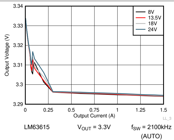
图 8-19. 线性和负载调整率
