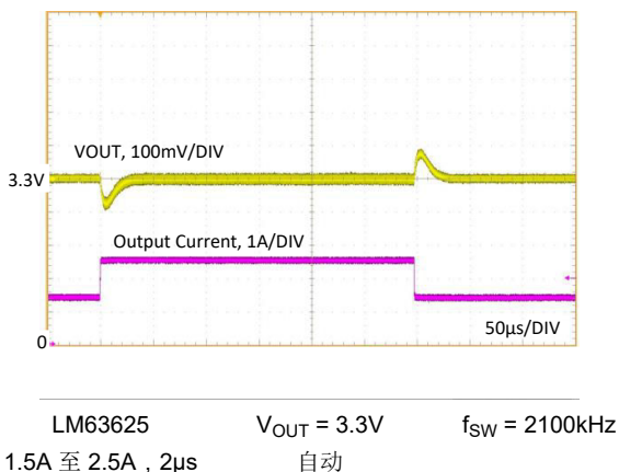
图 8-30. 负载瞬态
