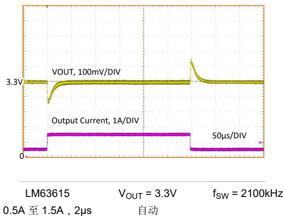
图 8-31. 负载瞬态
