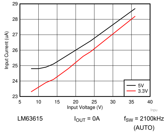
图 8-39. 输入电源电流与输入电压间的关系
