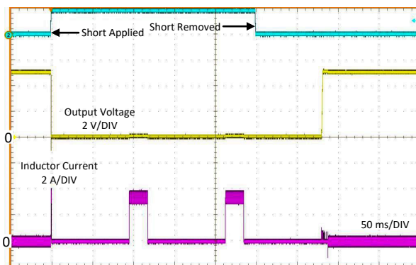
图 7-11. 短路瞬态和恢复；请参阅 LM63615/25 数据表
