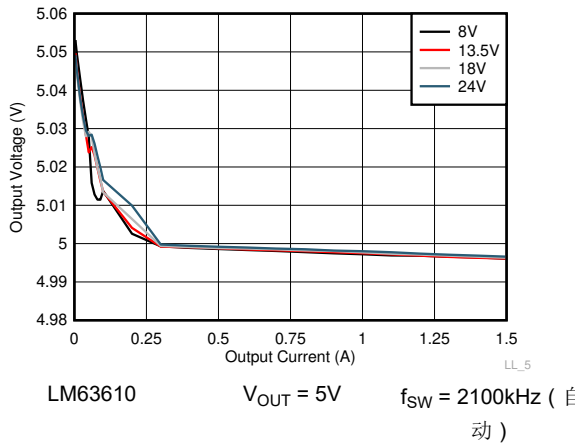
图 8-9. 线性和负载调整率
