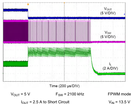
图 10-20. LM62440-Q1 Short Circuit Protection
