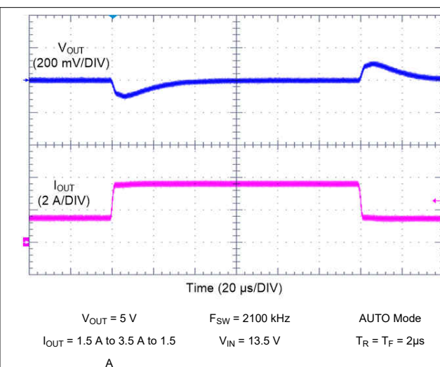
图 9-24. LM62435-Q1 Load Transient
