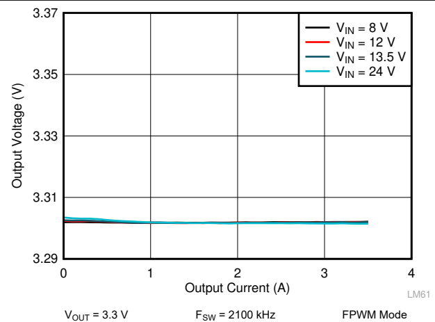
图 9-10. LM62435-Q1 Load and Line Regulation
