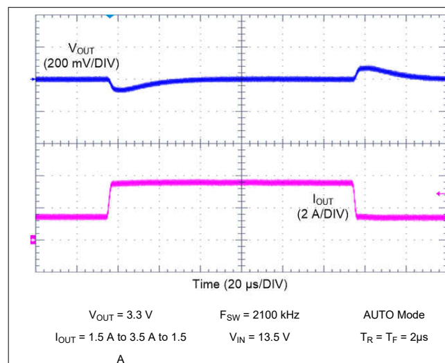
图 9-23. LM62435-Q1 Load Transient
