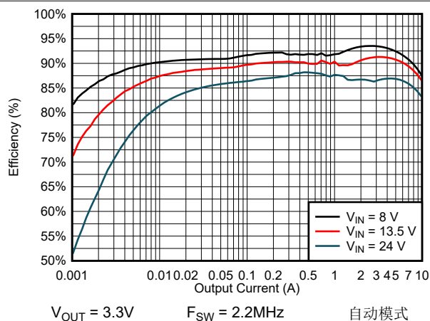
图 8-9. 效率
