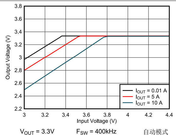
图 8-20. 压降
