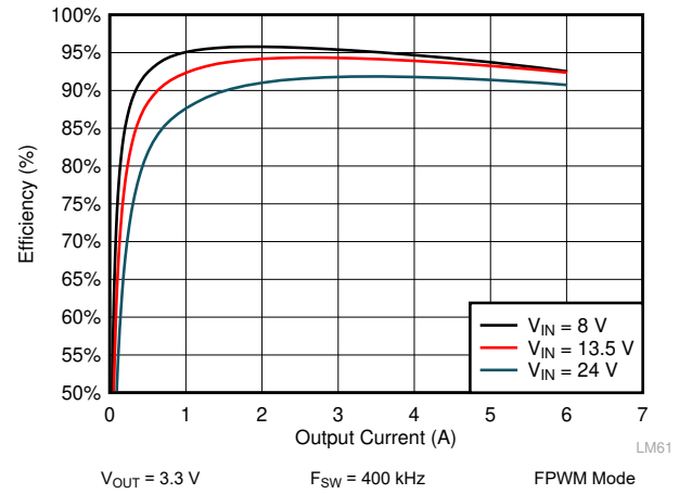
图 10-6. LM61460-Q1 Efficiency
