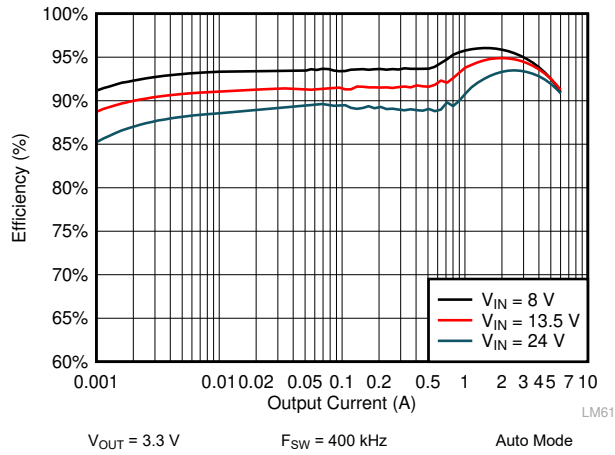
图 10-5. LM61460-Q1 Efficiency
