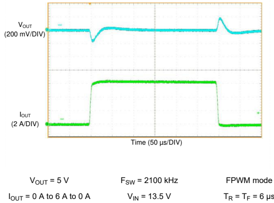
图 9-53. LM61460 Load Transient
