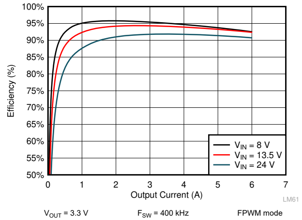
图 9-6. LM61460 Efficiency
