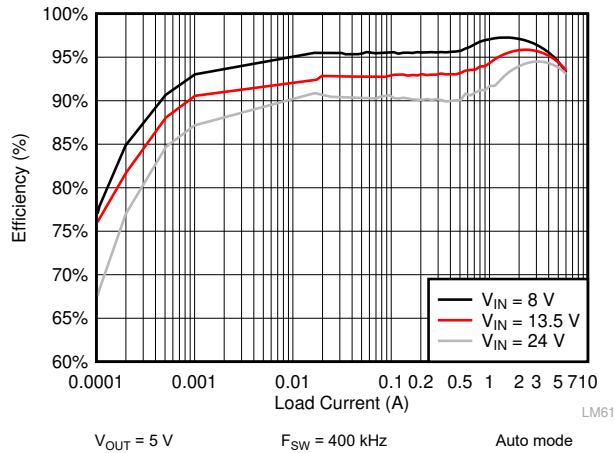
图 9-11. LM61460 Efficiency
