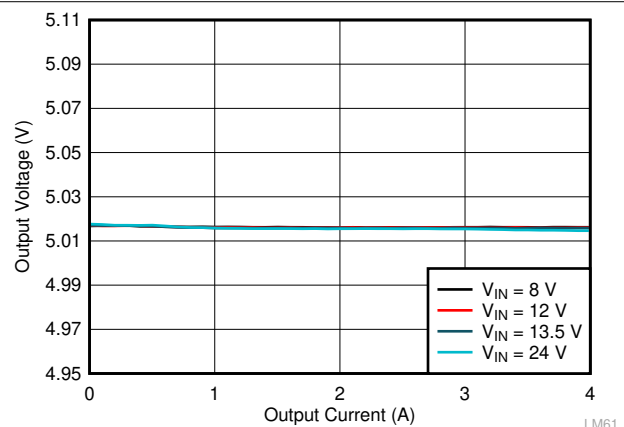
图 10-14. LM61440-Q1 Load and Line Regulation
