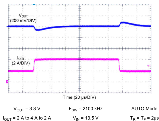
图 9-31. LM61440 Load Transient
