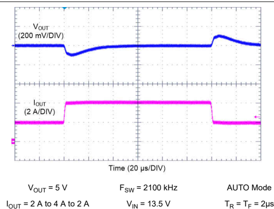
图 9-32. LM61440 Load Transient
