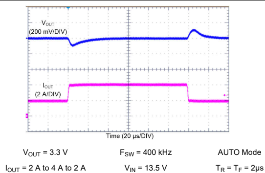
图 9-30. LM61440 Load Transient
