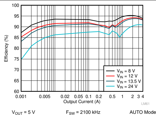
图 9-6. LM61440 Efficiency
