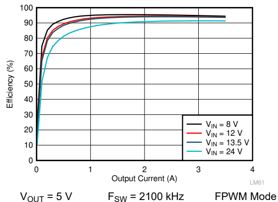
图 9-8. LM61435-Q1 Efficiency
