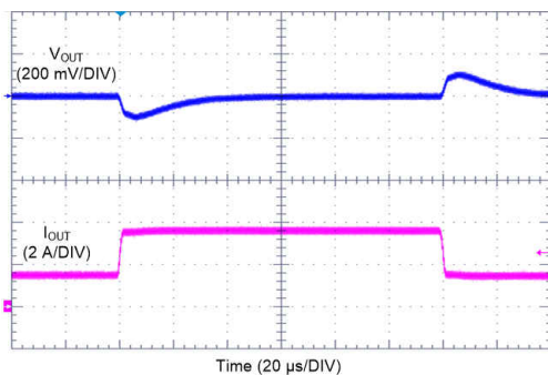
图 9-31. LM61435-Q1 Load Transient
