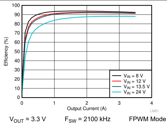
图 9-6. LM61435-Q1 Efficiency
