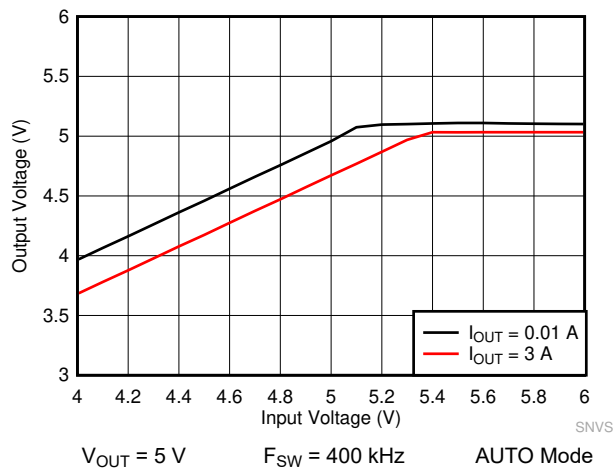
图 9-19. LM61435-Q1 Dropout Curve
