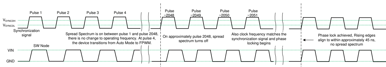
图 8-4. Synchronization Process
