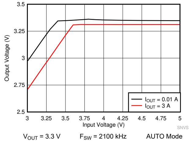
图 9-18. LM61435-Q1 Dropout Curve
