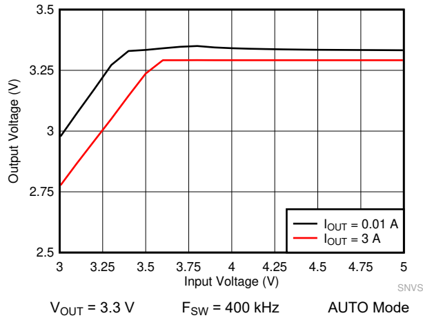
图 9-17. LM61435-Q1 Dropout Curve
