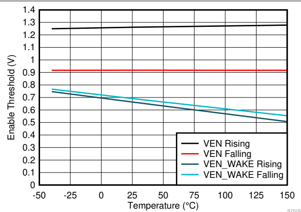
图 7-7. Enable Thresholds
