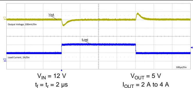
图 16. Load Transient
