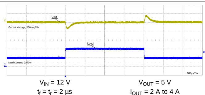
图 16. Load Transient
