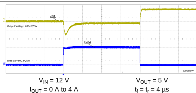
图 15. Load Transient
