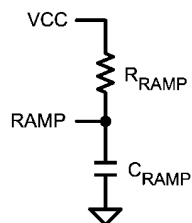
图7: R_{\text{RAMP}} 和 V_{\text{CC}} 图示 ( V_{\text{OUT}} > 7.5\text{V} 时)
