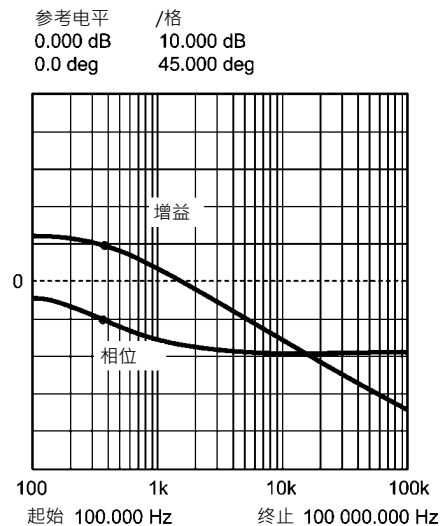
图9:调制器的增益和相位 R_{LOAD} = 5\Omega ， C_{OUT} = 130\mu F
