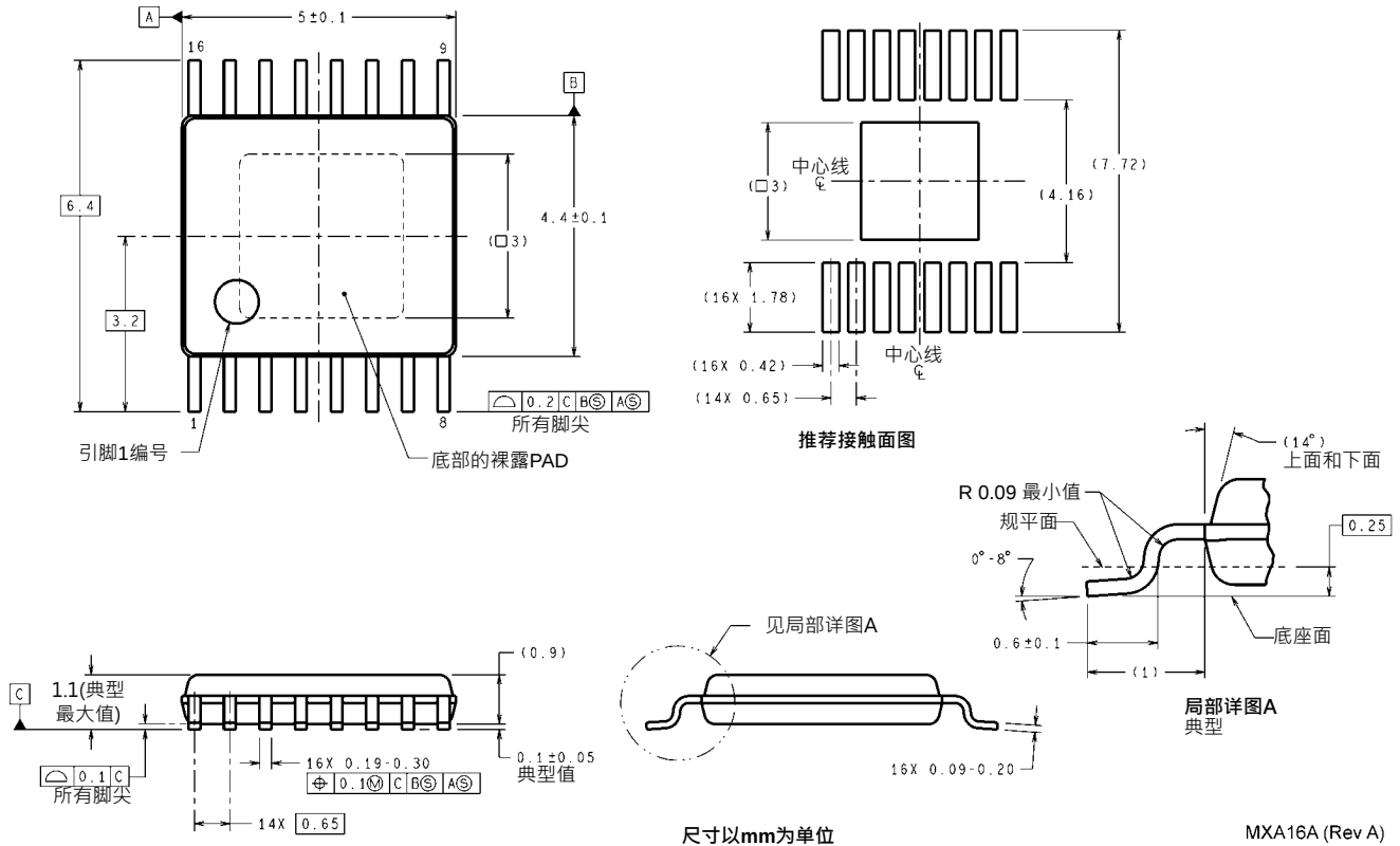
16引脚TSSOP封装 NS封装号MXA16A
