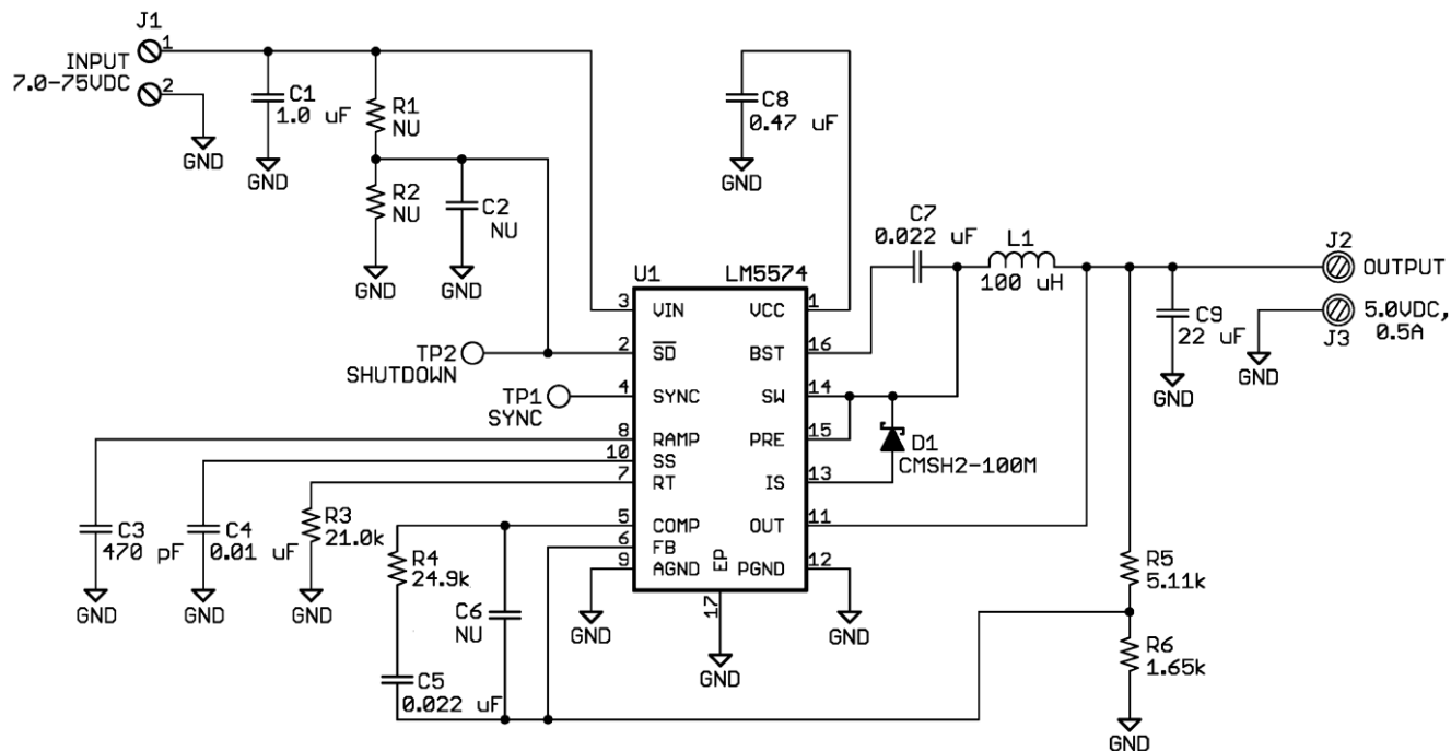
图 7-1. LM5574 Reference Schematic
