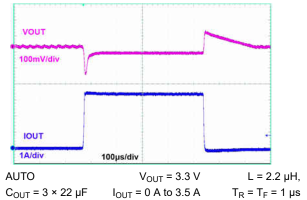
图 9-30. Load Transient
