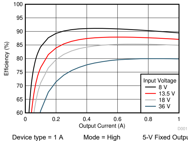
图 9-4. Efficiency
