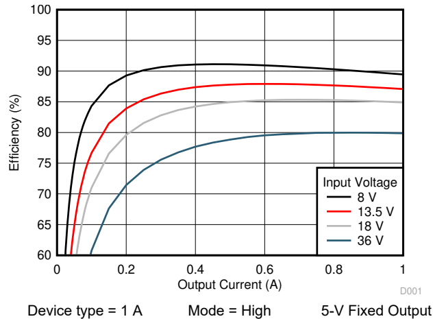
图 9-4. Efficiency
