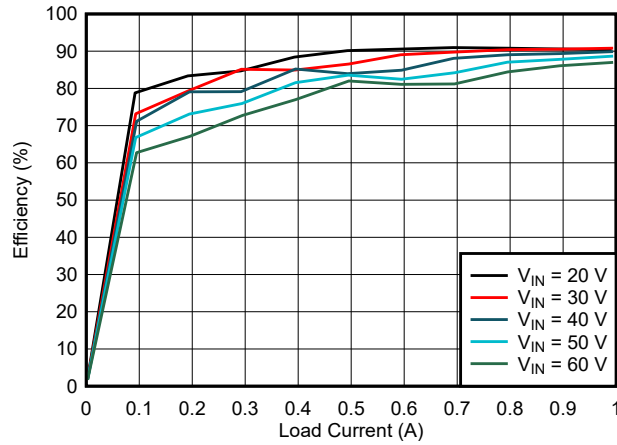
图 6-1. 效率与负载间的关系
