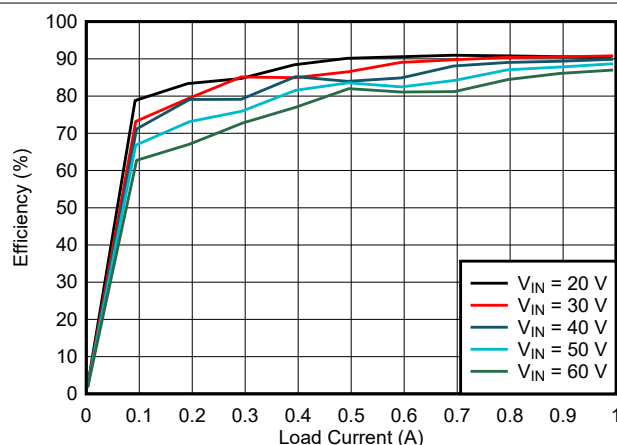
图 8-2. 效率
