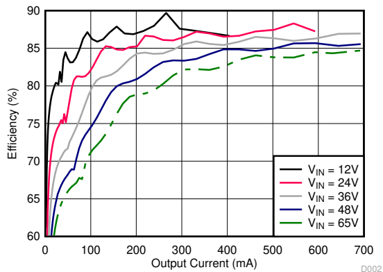
图 9-2. Efficiency (Linear Scale)
