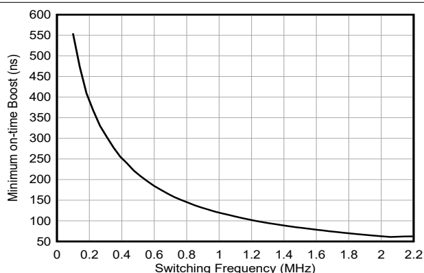
图 5-21. 升压最短导通时间与开关频率间的关系
