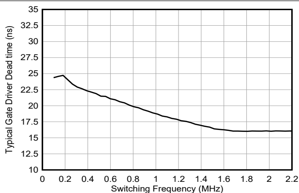
图 5-23. 栅极驱动器转换 (死区) 时间与开关频率间的关系 SEL_MIN_DEADTIME_GDRV = 0b01, SEL_SCALE_DT = 0b0, EN_CONST_TDEAD = 0b0
