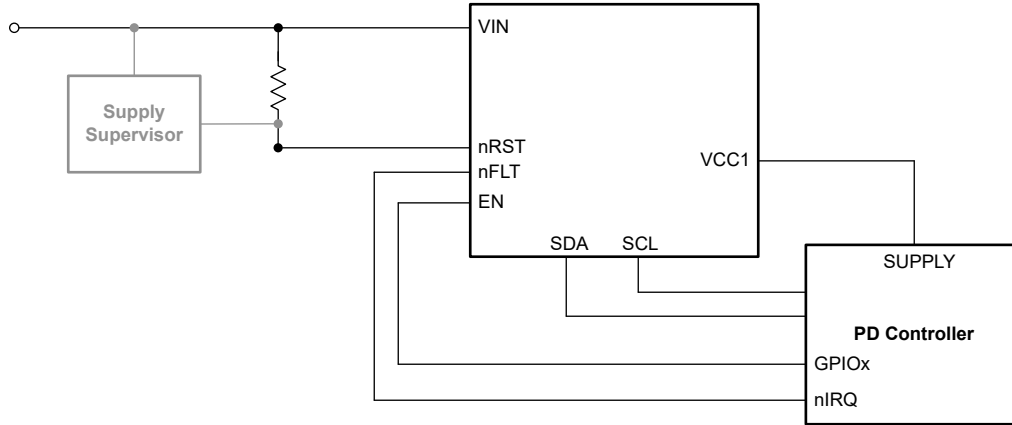
图 7-15. 简化版原理图
