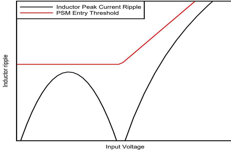
图 7-9. PSM 进入阈值与纹波电流随输入电压变化的通用曲线图
