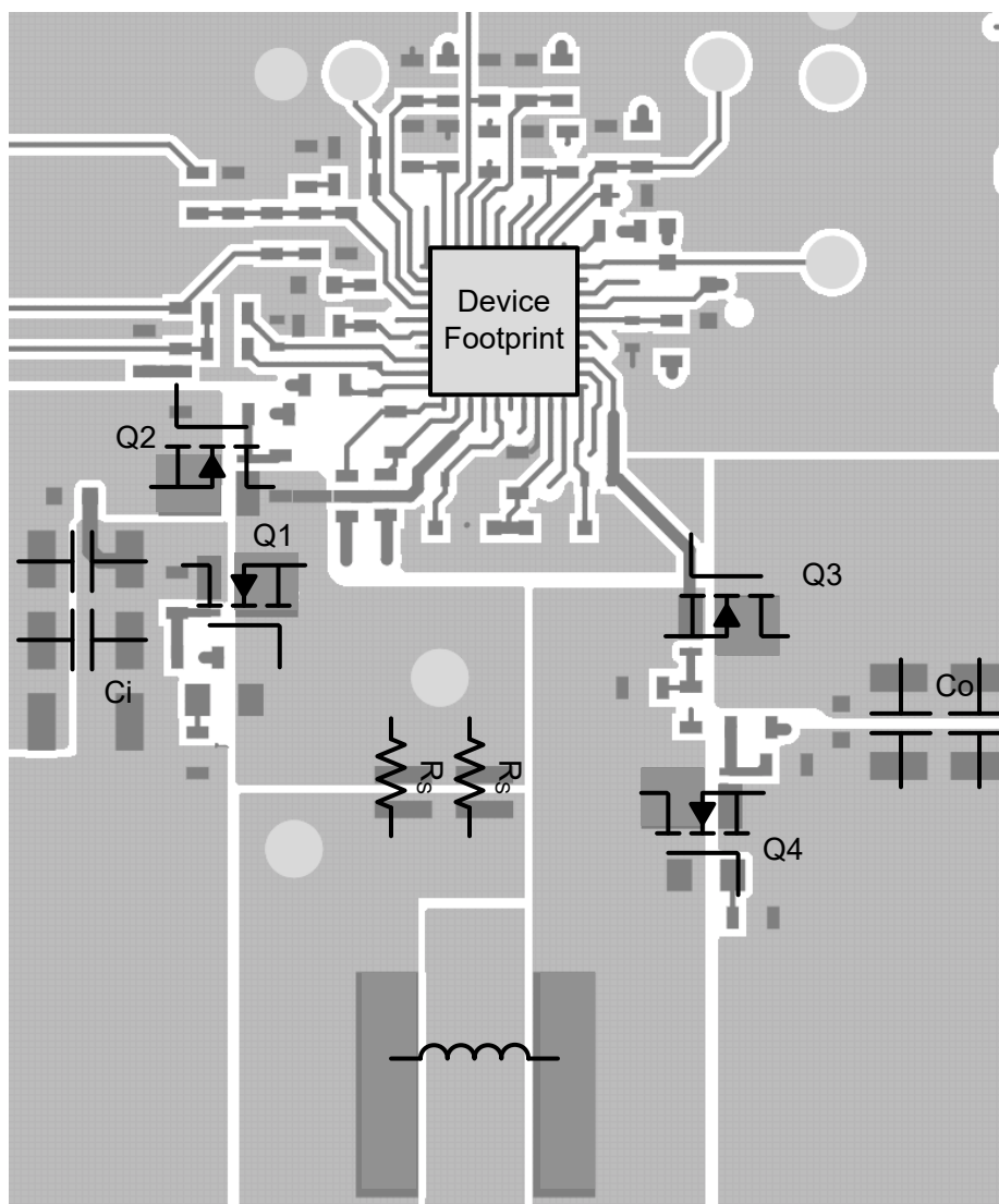
图 9-31. LM51772-Q1 简化版顶层示例
