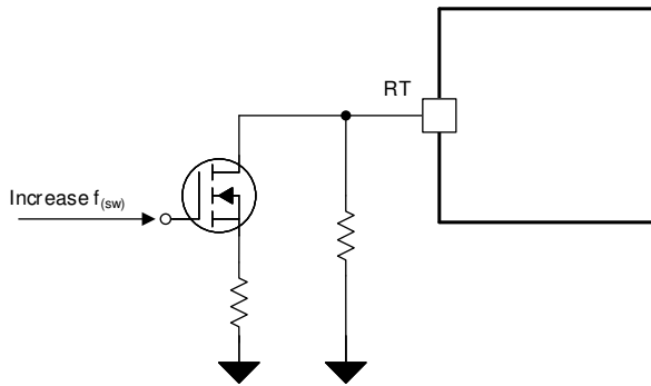
图 7-23. 跳频示例
