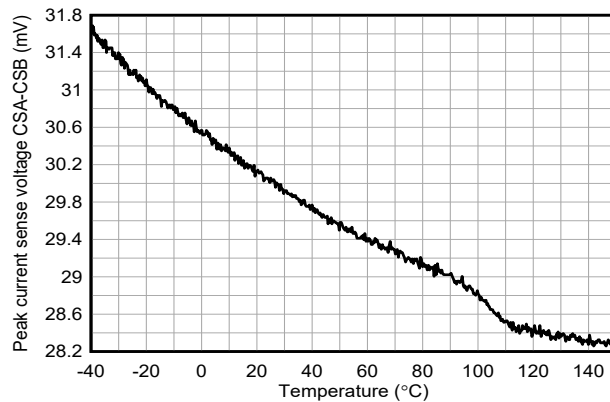
图 5-29. 平均电流限制阈值电压与温度间的关系 ILIM_THRESHOLD = 0x3C
