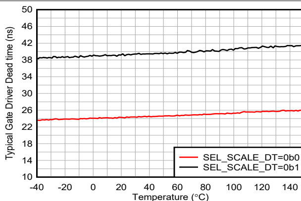
图 5-24. 栅极驱动器转换 (死区) 时间与开关频率间的关系 f_{(sw)} = 100\text{kHz} , SEL_MIN_DEADTIME_GDRV = 0b01, EN_CONST_TDEAD = 0b0, 低侧关断, 高侧导通
