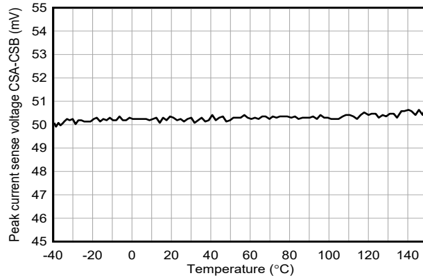
图 5-25. 峰值电流限制阈值电压与温度间的关系
