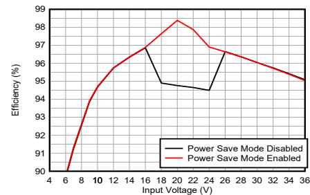
效率与输入电压间的关系, V_O = 20\text{V} , I_O = 5\text{A}
