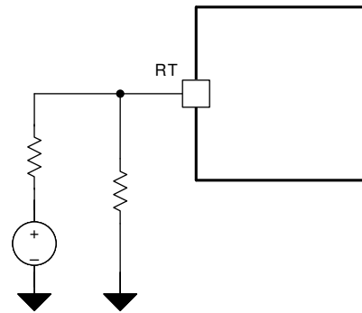
图 7-24. 动态更改频率的示例
