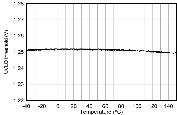
图 5-16. EN/UVLO 阈值与温度间的关系
