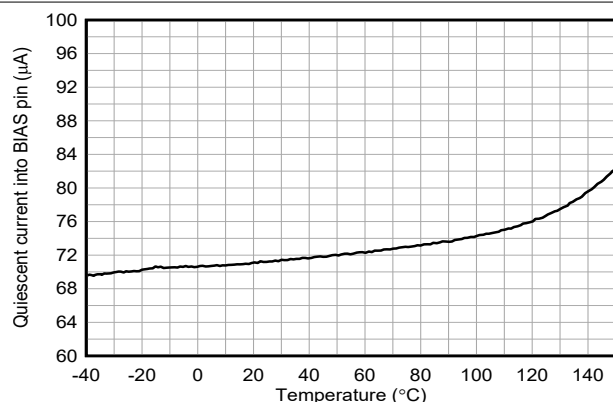
图 5-9. 流入 BIAS 的静态电流与 BIAS 间的关系 V_{(BIAS)} = 12\text{V} , V_{(VIN)} = 3.5\text{V}
