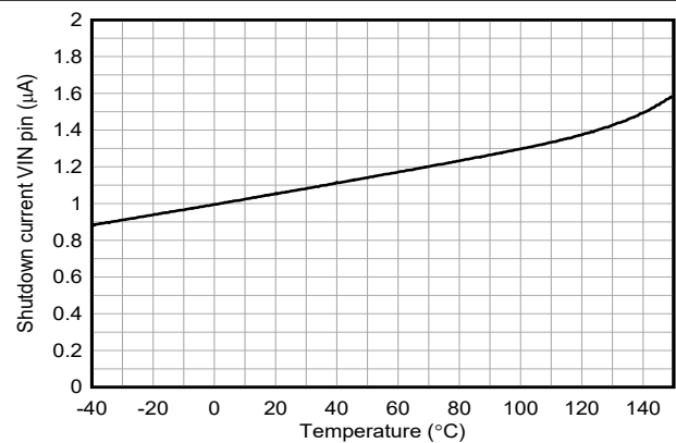
图 5-6. 流入 VIN 的关断电流与温度间的关系 V_{EN/UVLO} = 0\text{V} , V_{(VIN)} = 12\text{V} , V_{(BIAS)} = 0\text{V}
