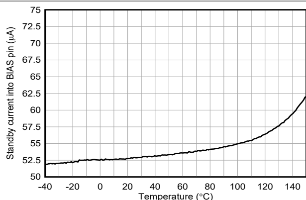
图 5-10. 流入 BIAS 的待机电流与温度间的关系 V_{(VIN)} = 3.5\text{V} , V_{(VIN)} = 12\text{V}
