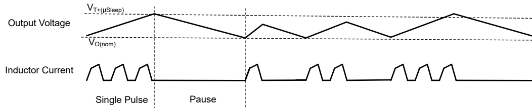
图 7-6. 省电模式的时序图 ( \mu Sleep 禁用 )
