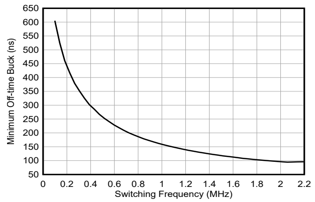
图 5-18. 降压最短关断时间与开关频率间的关系
