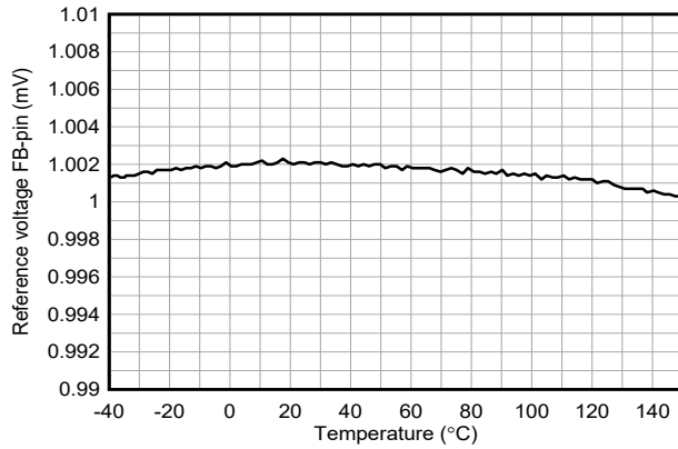
图 5-3. FB 引脚基准电压与温度间的关系
