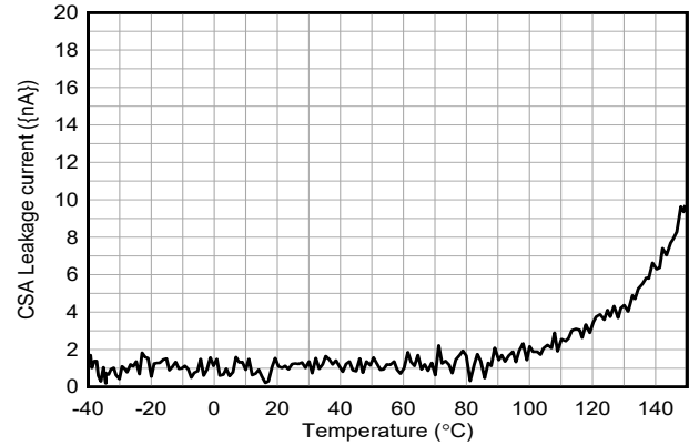
图 5-26. CSA 输入电流与温度间的关系
