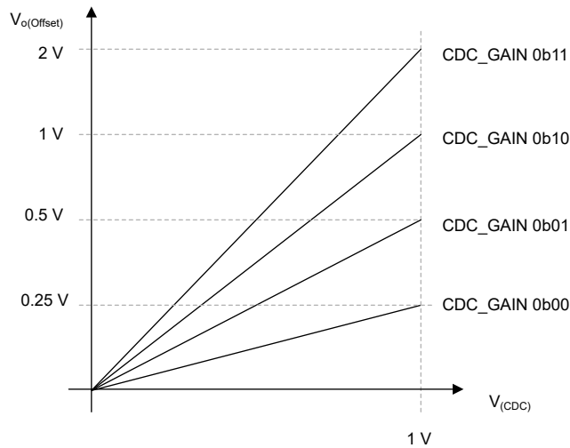
图 7-31. Vo 偏移电压与 CDC 电压的关系
