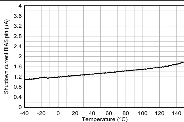
图 5-7. 流入 BIAS 的关断电流与温度间的关系 V_{EN/UVLO} = 0\text{V} , V_{(VIN)} = 3.5\text{V} , V_{(BIAS)} = 12\text{V}
