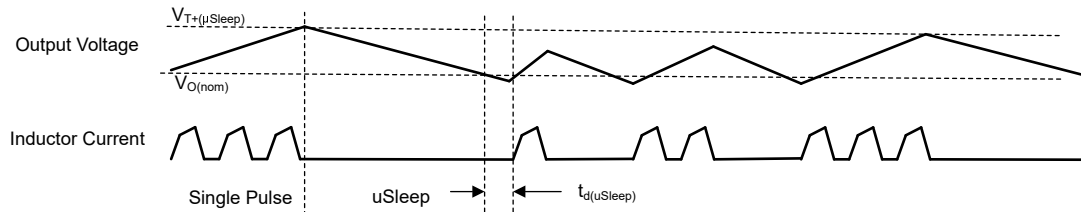
图 7-7. 省电模式的时序图 ( \mu Sleep 启用 )
