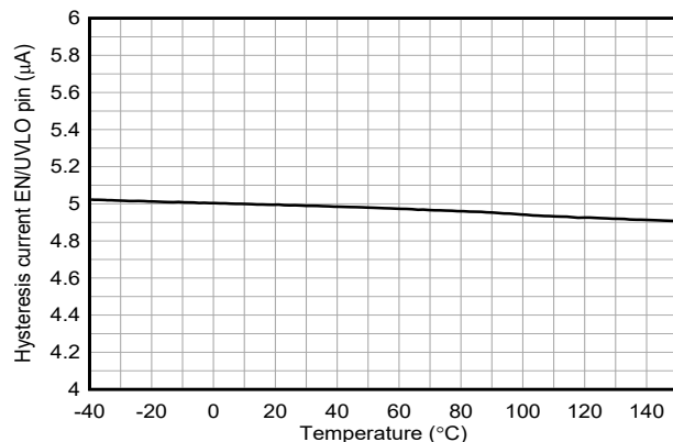
图 5-17. EN/UVLO 上的迟滞电流与温度间的关系
