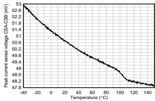
图 5-28. 平均电流限制阈值电压与温度间的关系 ILIM_THRESHOLD = 0x64
