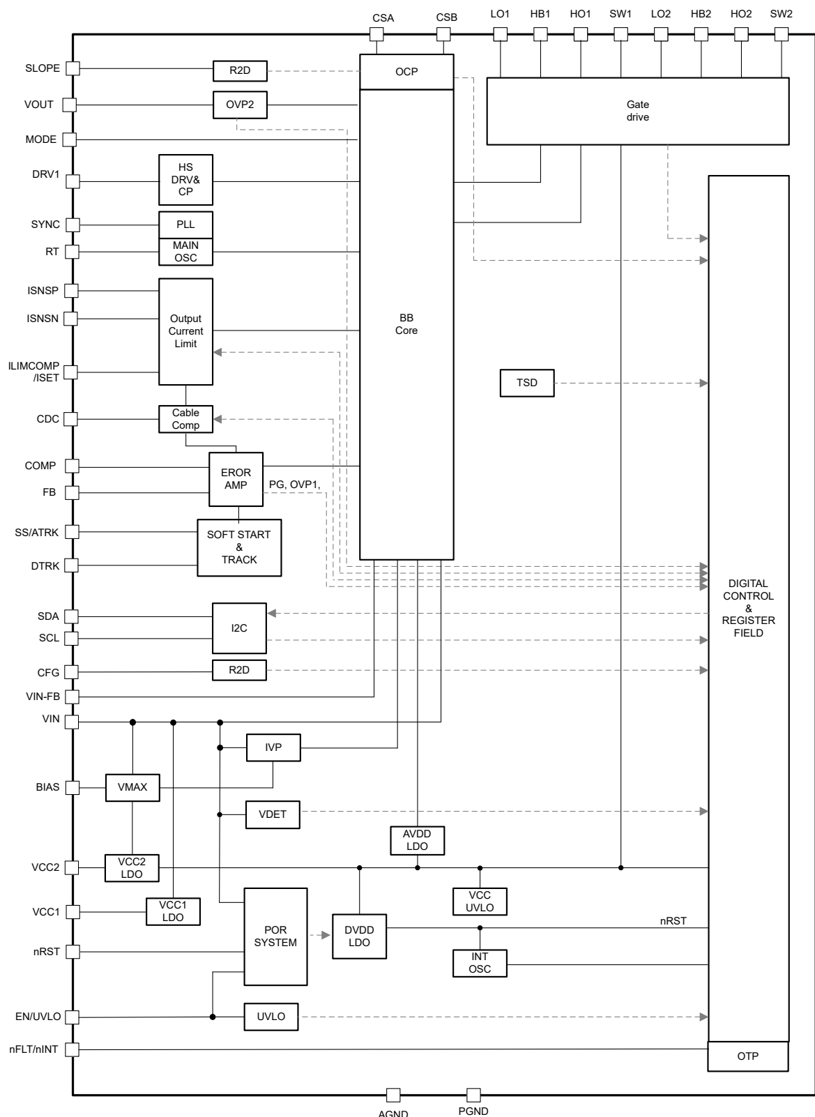
图 7-1. LM51772-Q1 功能方框图
