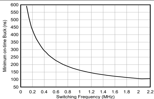
图 5-19. 降压最短导通时间与开关频率间的关系
