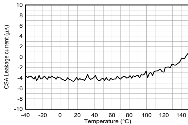
图 5-27. CSB 输入电流与温度间的关系
