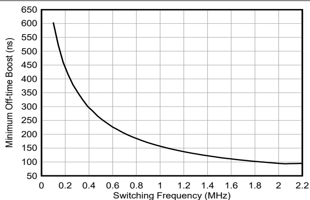
图 5-20. 升压最短关断时间与开关频率间的关系
