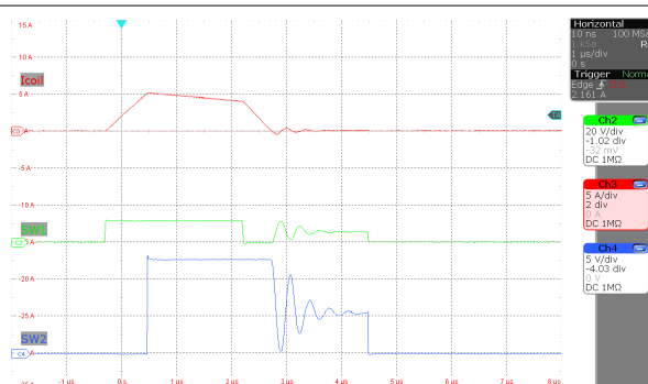
图 9-7. 电感器电流降压/升压操作 ( \text{MODE} = 0\text{V} , V_o = 12\text{V} , I_o = 10\text{mA} , V_{(\text{VIN})} = 12\text{V} )
