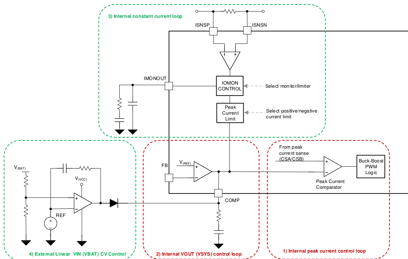
图 9-17. 直流/直流备用应用的控制环路概述
