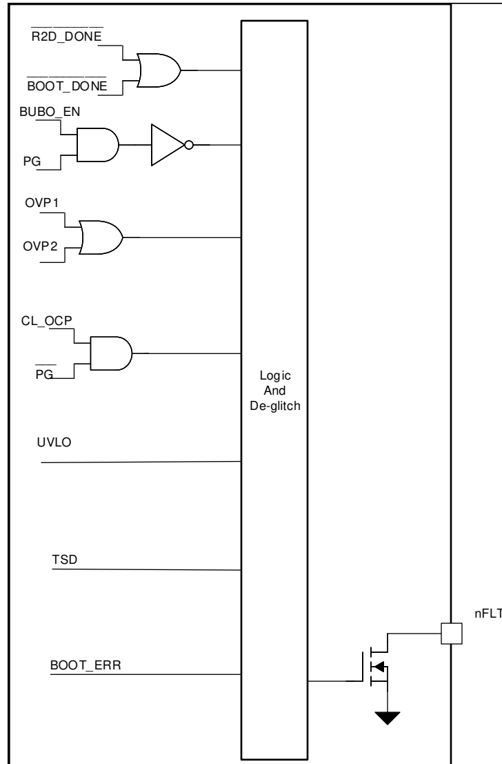
图 8-19. nFLT 引脚逻辑功能方框图
