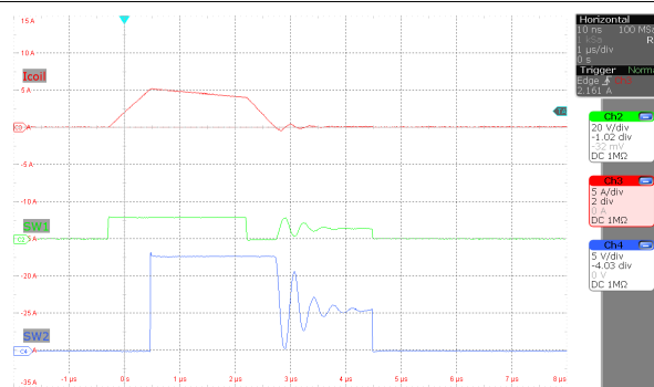
图 8-7. 电感器电流降压/升压操作 ( MODE = 0V , V_o = 12V , I_o = 10mA , V_{(VIN)} = 12V )
