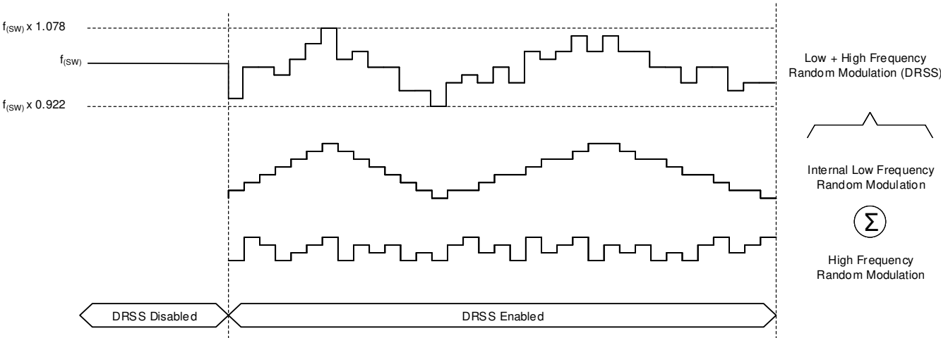
图 7-18. 双随机展频
