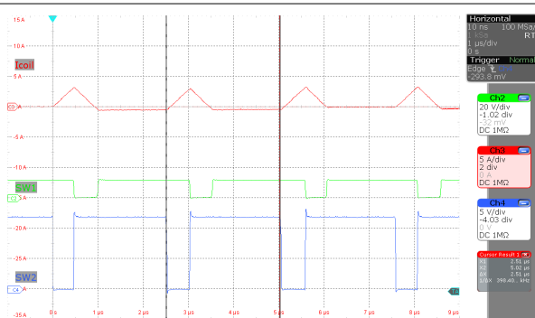
图 8-4. 电感器电流降压/升压操作 ( MODE = V_{(VCC)} , V_o = 12V , I_o = 0A , V_{(VIN)} = 12V )
