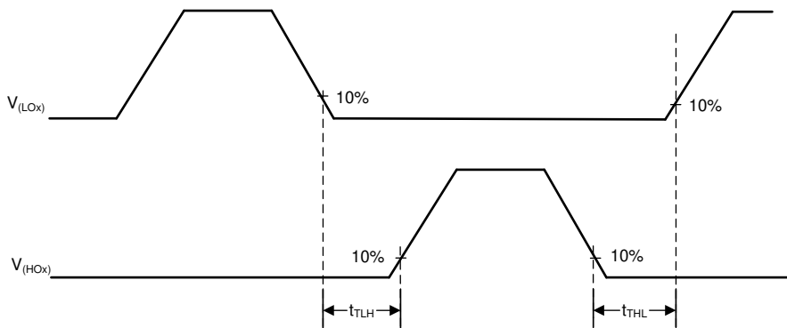
图 6-2. 栅极驱动器时序图, t_d
