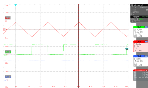
图 8-5. 电感器电流降压操作 ( MODE = V_{(VCC)} , V_o = 12V , I_o = 0A , V_{(VIN)} = 24V )
