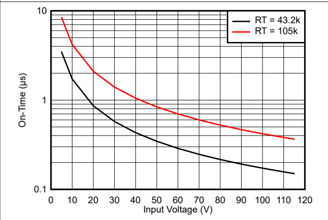
图 7-4. COT On Time Versus Input Voltage
