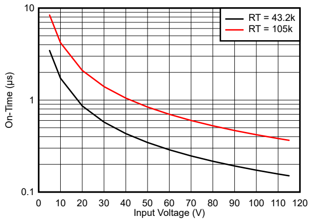
图 6-4. COT On Time Versus Input Voltage
