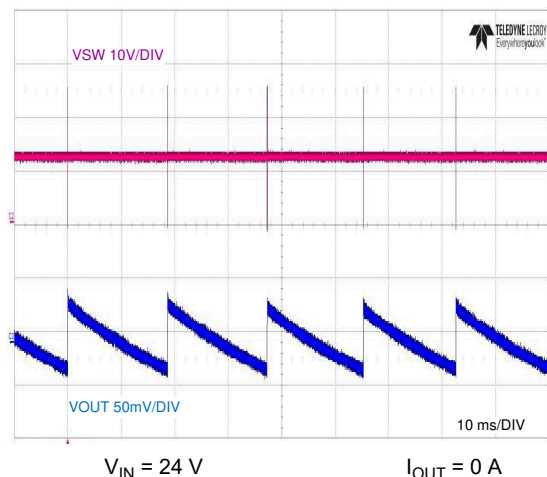
图 8-14. No-Load Switching
