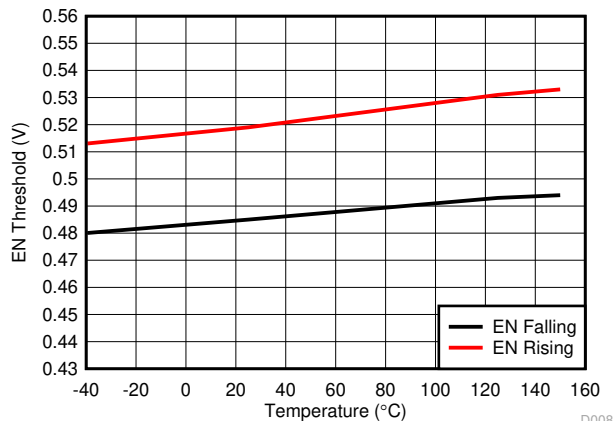
图 8-8. EN 阈值与温度间的关系
