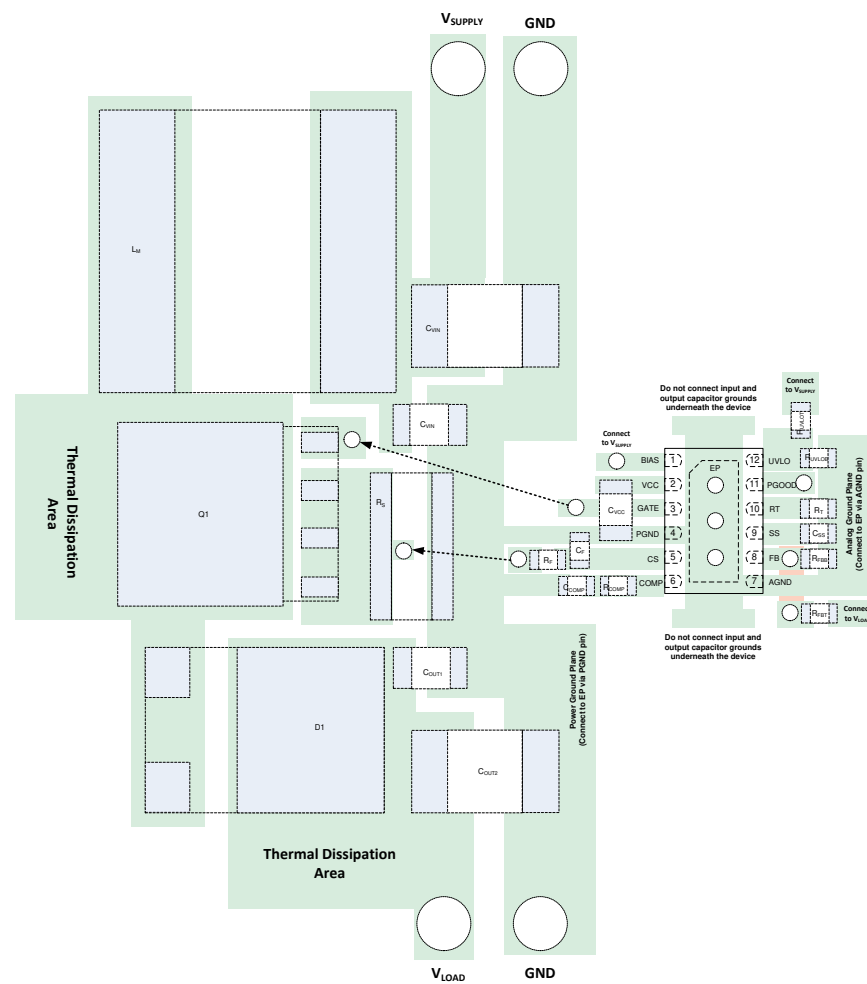
图 12-1. PCB 布局示例 1
