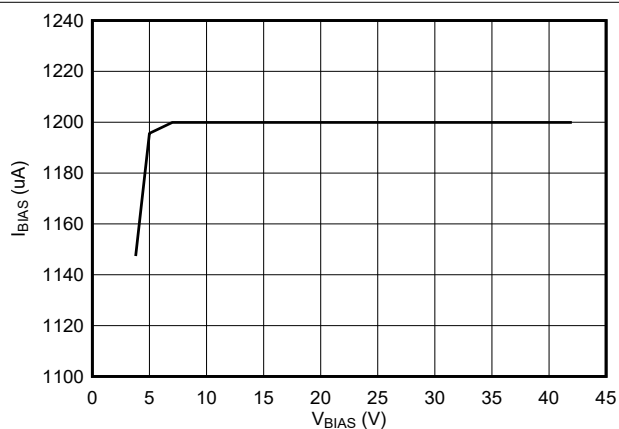
图 8-4. VBIAS vs IBIAS (Active Mode)
