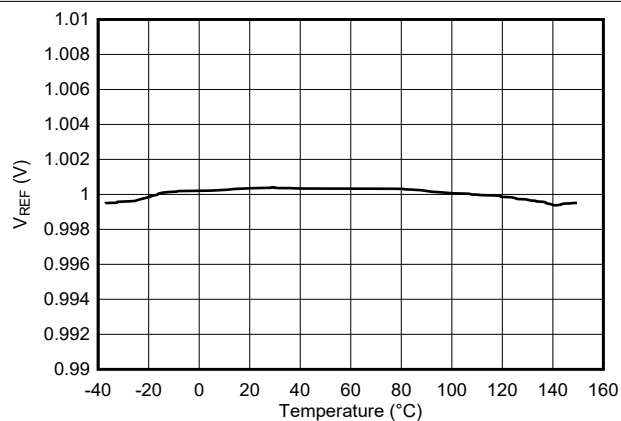
图 8-16. V_{REF} vs Temperature
