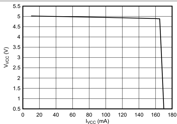
图 8-9. V_{VCC} vs I_{VCC}
