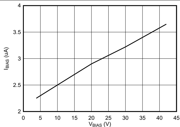
图 8-7. V_{BIAS} vs I_{BIAS} (Shutdown Mode)
