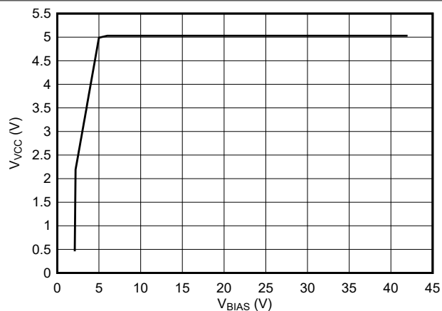
图 8-8. V_{BIAS} vs V_{VCC}
