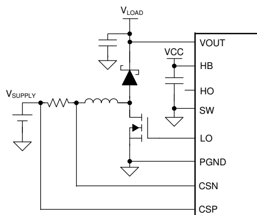
图 10-9. Non-Synchronous Boost Configuration
