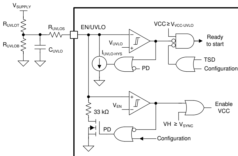
图 9-1. EN/UVLO Circuit
