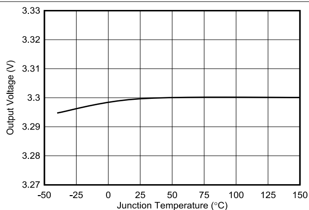
图 7-6. Fixed 3.3-V Output Voltage vs Temperature
