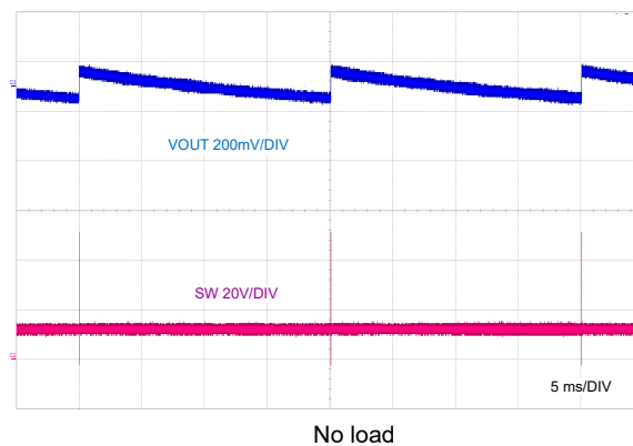
图 9-21. PFM Switching
