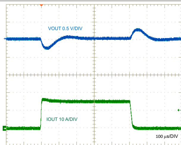
图 10-26. 负载瞬态，0A 至 15A
