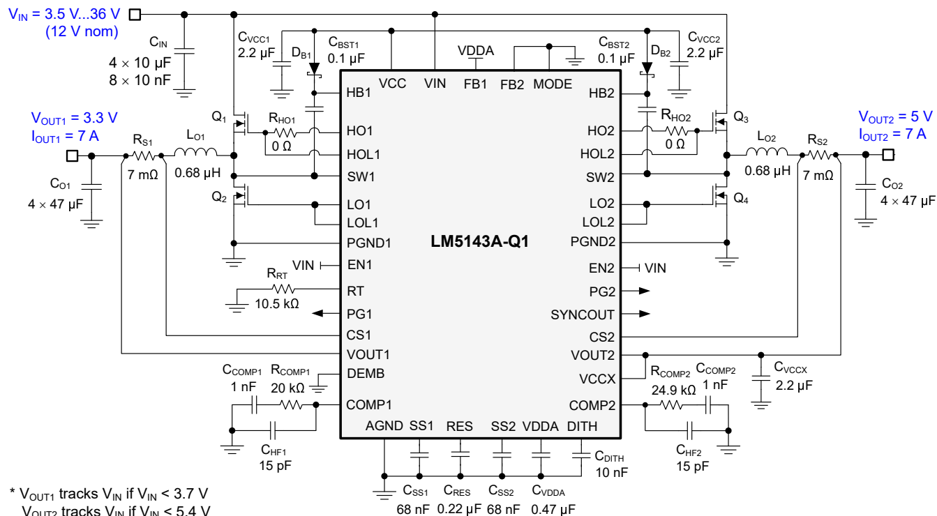
图 10-4. 采用 LM5143A-Q1 双路输出降压稳压器且开关频率为 2.1MHz 时的应用电路 1
