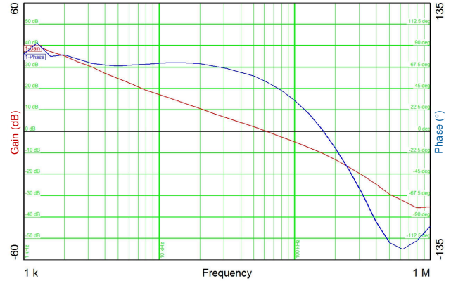
图 9-18. Bode Plot, 5-V Output
