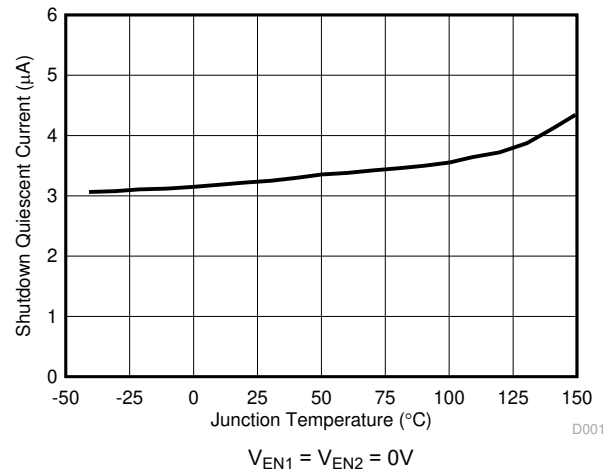
图 8-6. 关断电流与温度之间的关系
