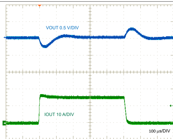
图 10-26. 负载瞬态，0A 至 15A
