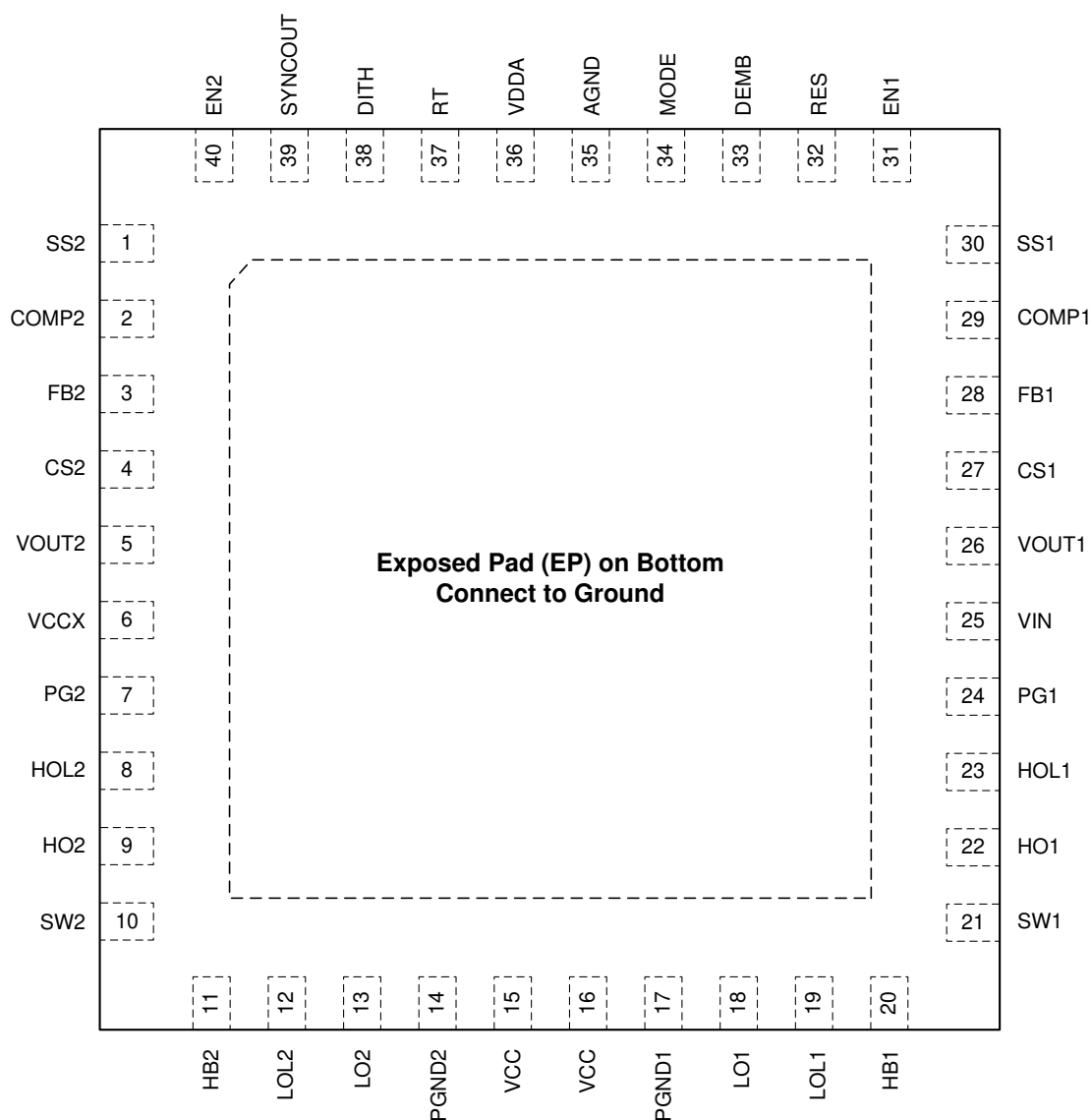
图 7-1. 40 引脚 VQFN RHA 封装 (顶视图)
