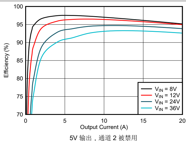
图 8-5. 效率与 I_{OUT1} 之间的关系
