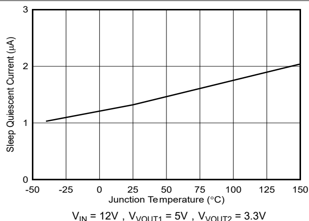
图 6-9. 睡眠静态电流与温度间的关系
