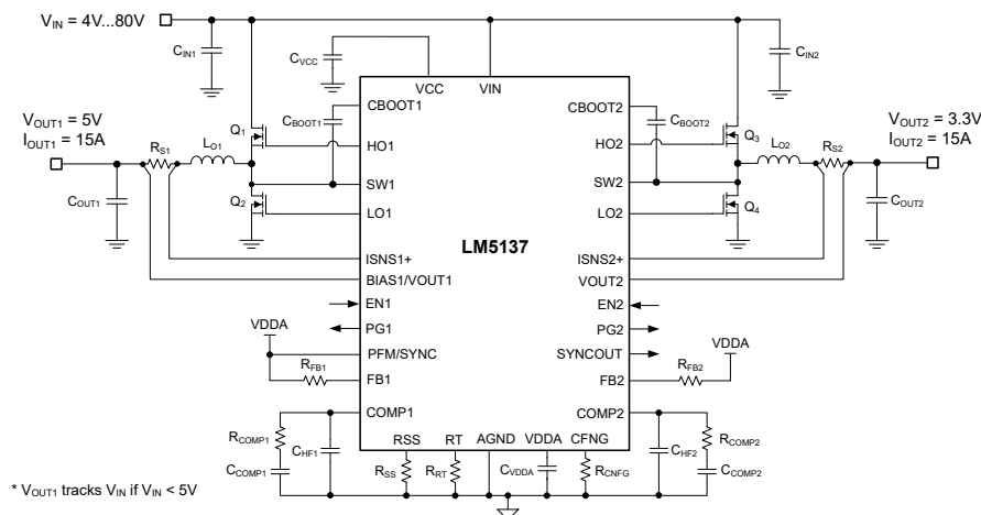
LM5137 双路输出降压开关稳压器 - 简化原理图
