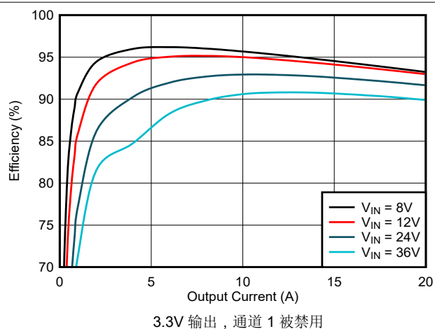
图 8-6. 效率与 I_{OUT2} 之间的关系
