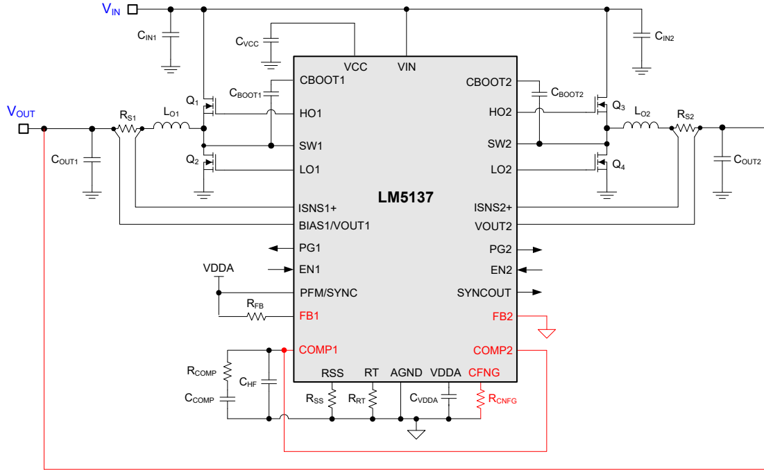
图 7-8. LM5137 配置为单输出交错式操作时的两相稳压器原理图
