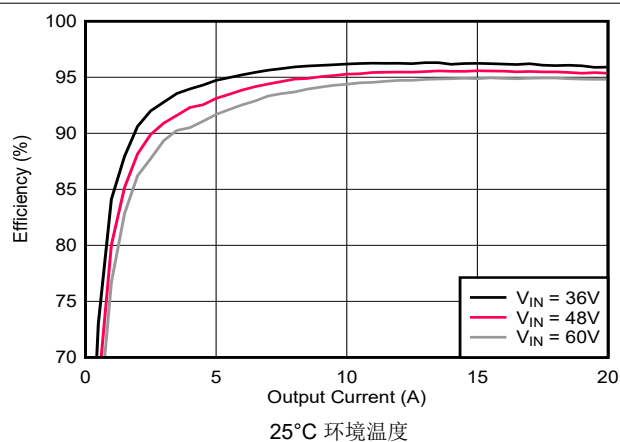
图 8-21. 效率与 I_{OUT} 间的关系，PFM/SYNC 连接至低电平
