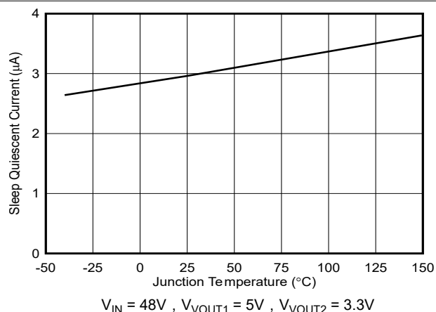
图 6-10. 睡眠静态电流与温度间的关系
