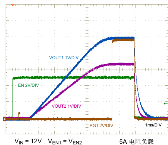
图 8-8. 使能端开启和关闭特性
