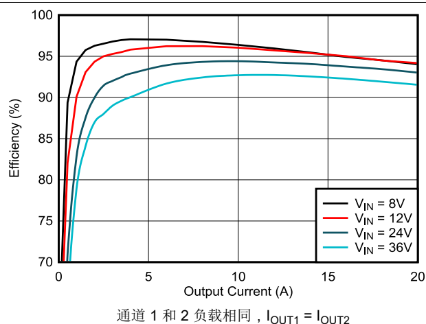
图 8-7. 效率与 I_{OUT} 之间的关系
