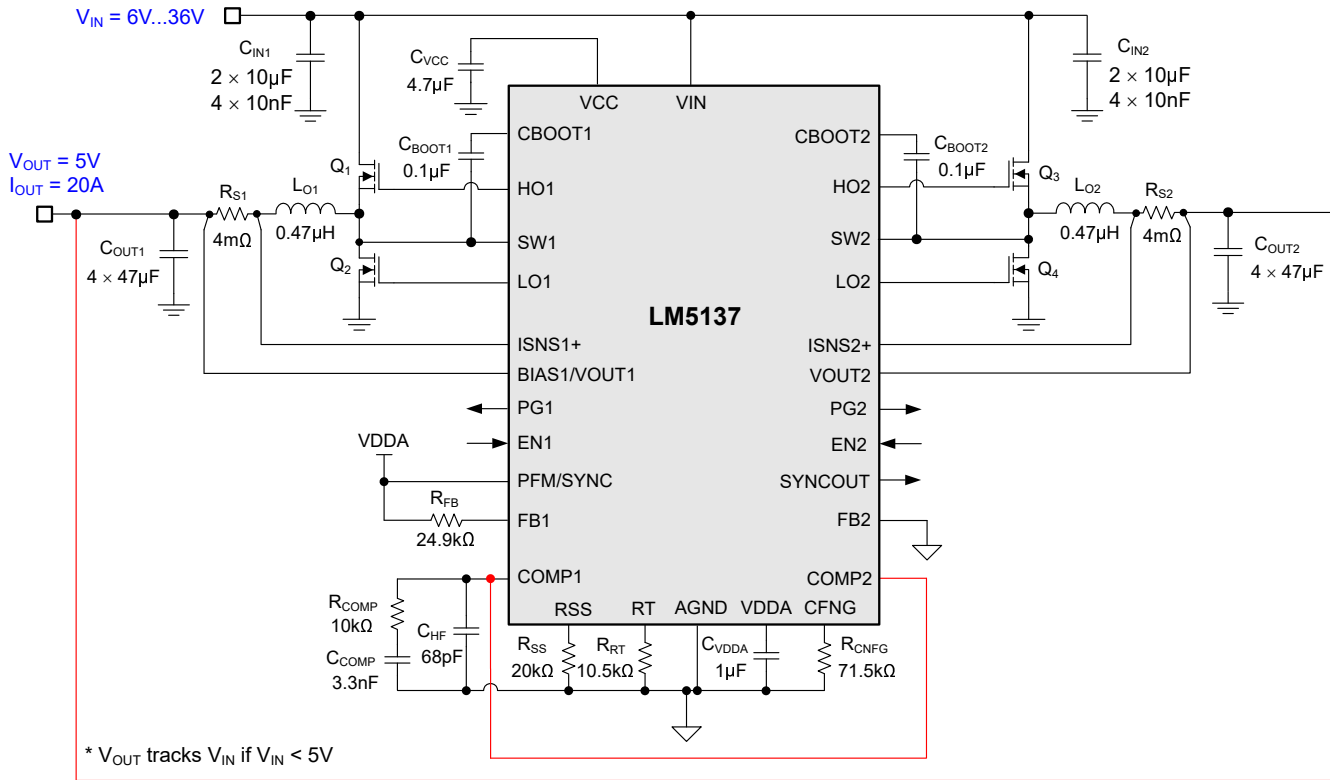
图 8-19. 采用 LM5137 两相降压稳压器且开关频率为 2.1MHz 时的应用电路 2
