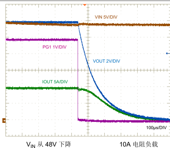
图 8-25. 关断特性
