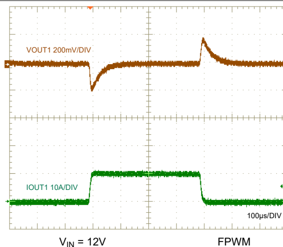
图 8-12. 负载瞬态，5V 输出，0A 至 10A
