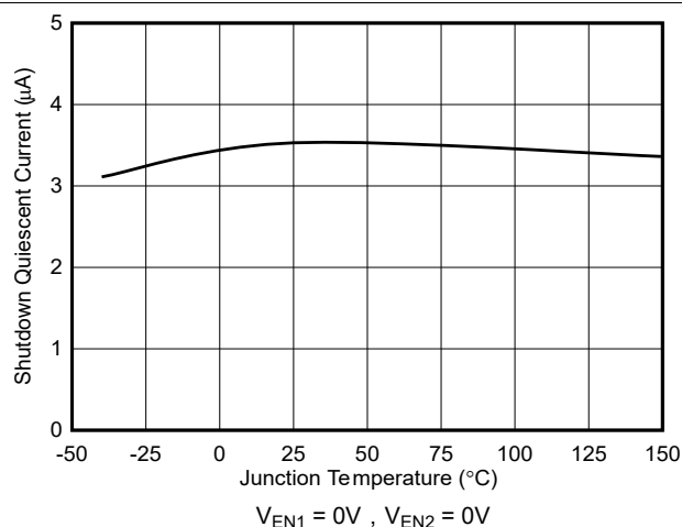
图 6-7. 关断静态电流与温度间的关系
