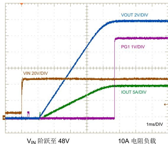
图 8-23. 启动特性
