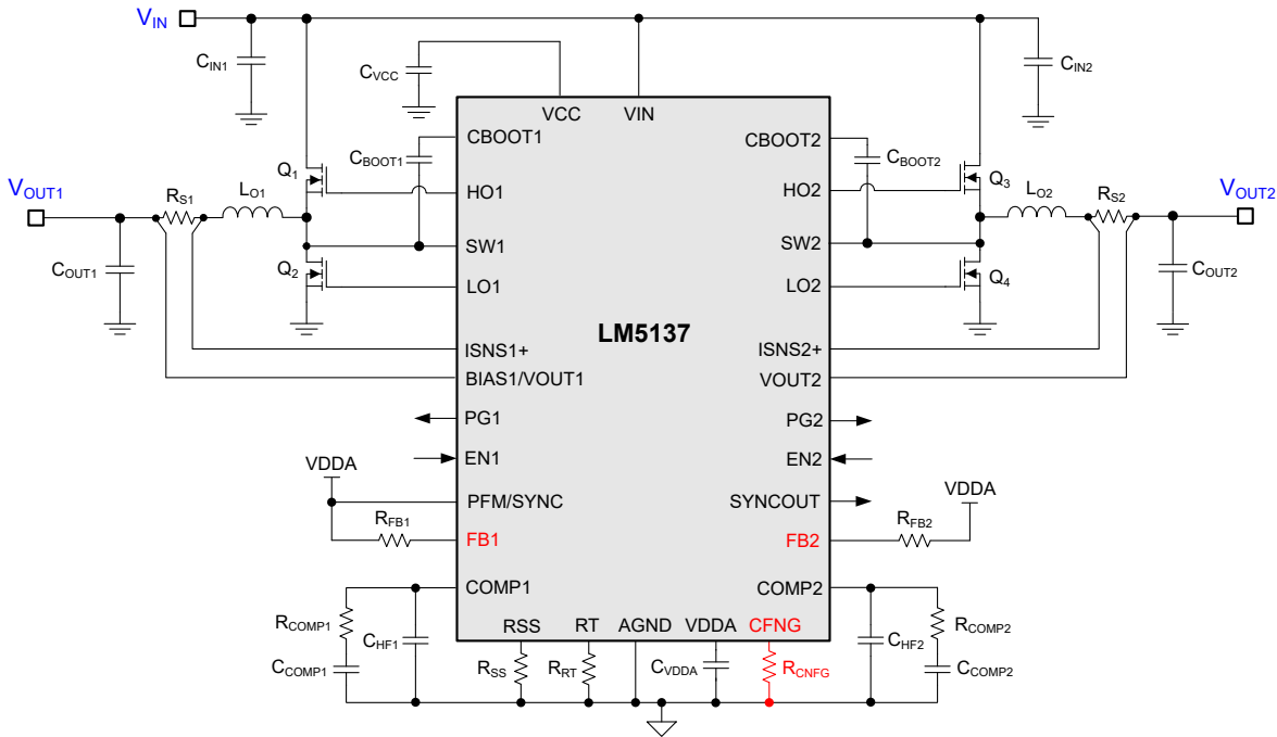
图 7-7. 为独立双路输出配置的 LM5137 稳压器原理图
