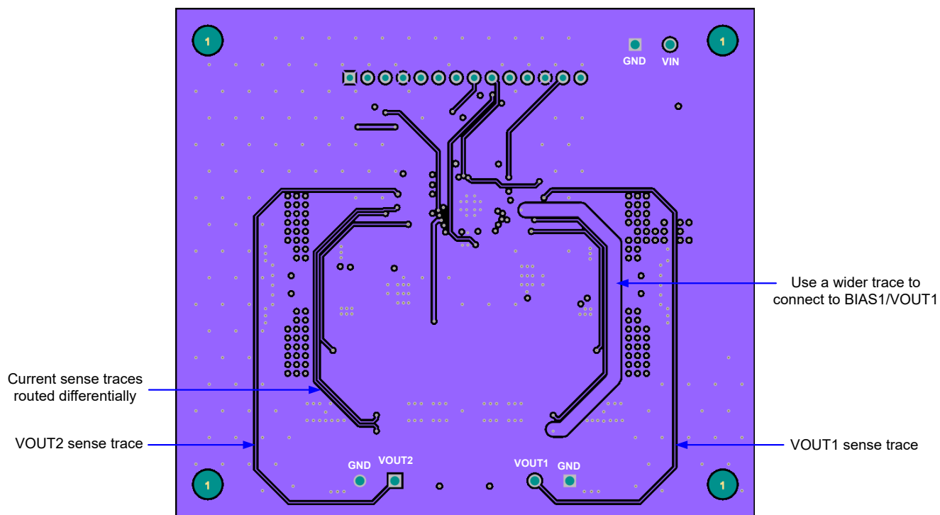
图 8-33. PCB 内层
