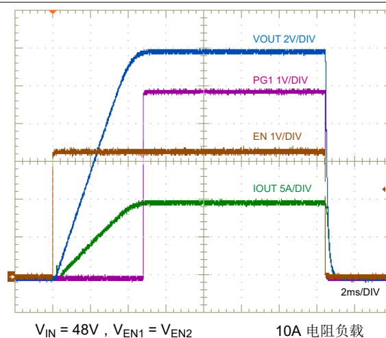
图 8-22. 使能端开启和关闭特性
