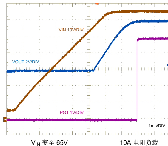
图 8-24. 预偏置启动特性
