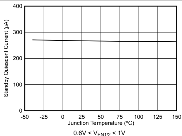
图 6-8. 待机静态电流与温度间的关系
