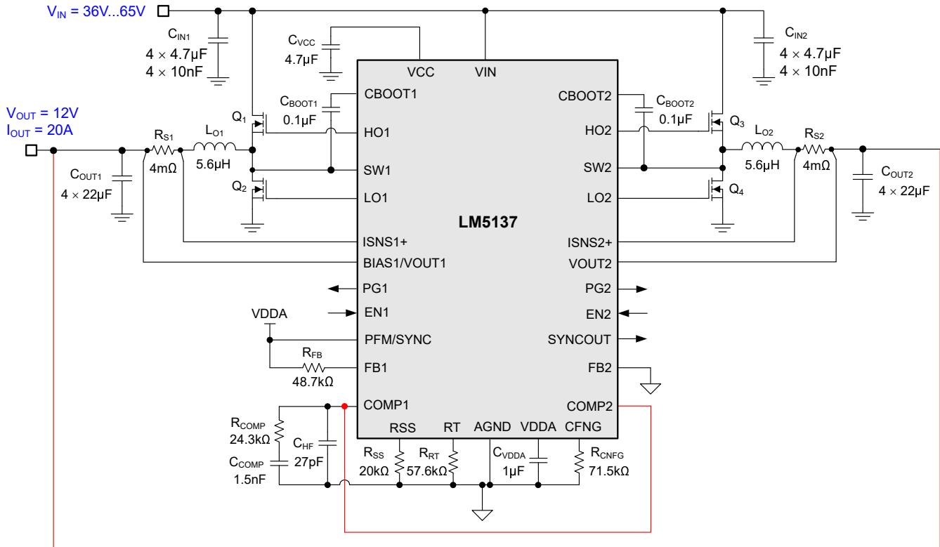
图 8-20. 采用 LM5137 两相降压稳压器且开关频率为 400kHz 时的应用电路 3
