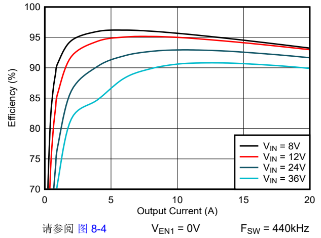
图 6-2. 效率与负载间的关系，3.3V 输出
