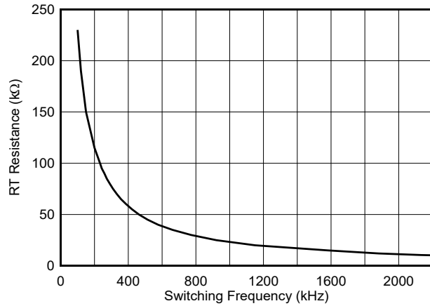
图 6-25. RT 电阻与开关频率间的关系
