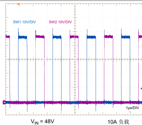
图 8-26. 开关节点电压
