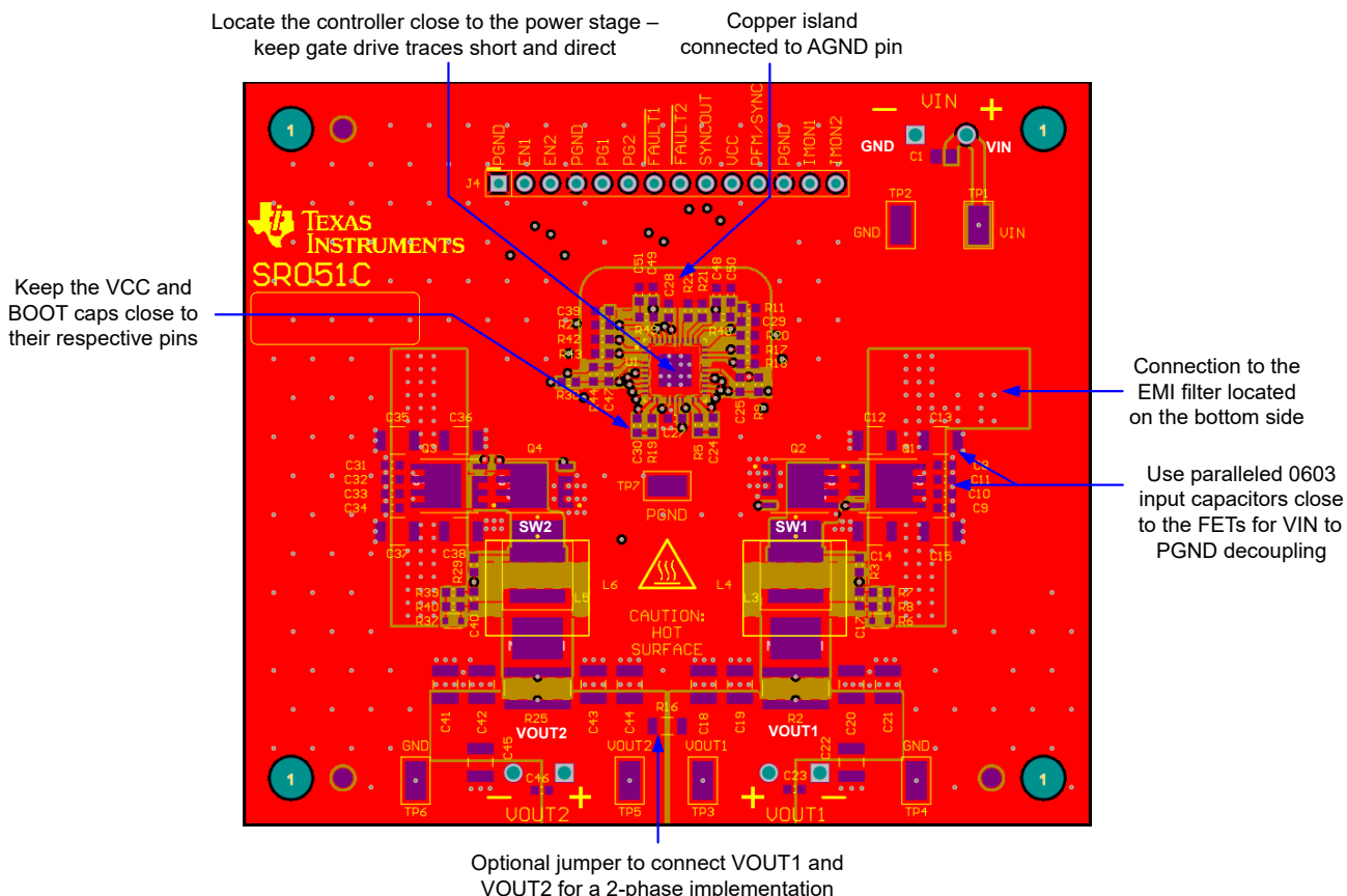
图 8-30. PCB 顶层
