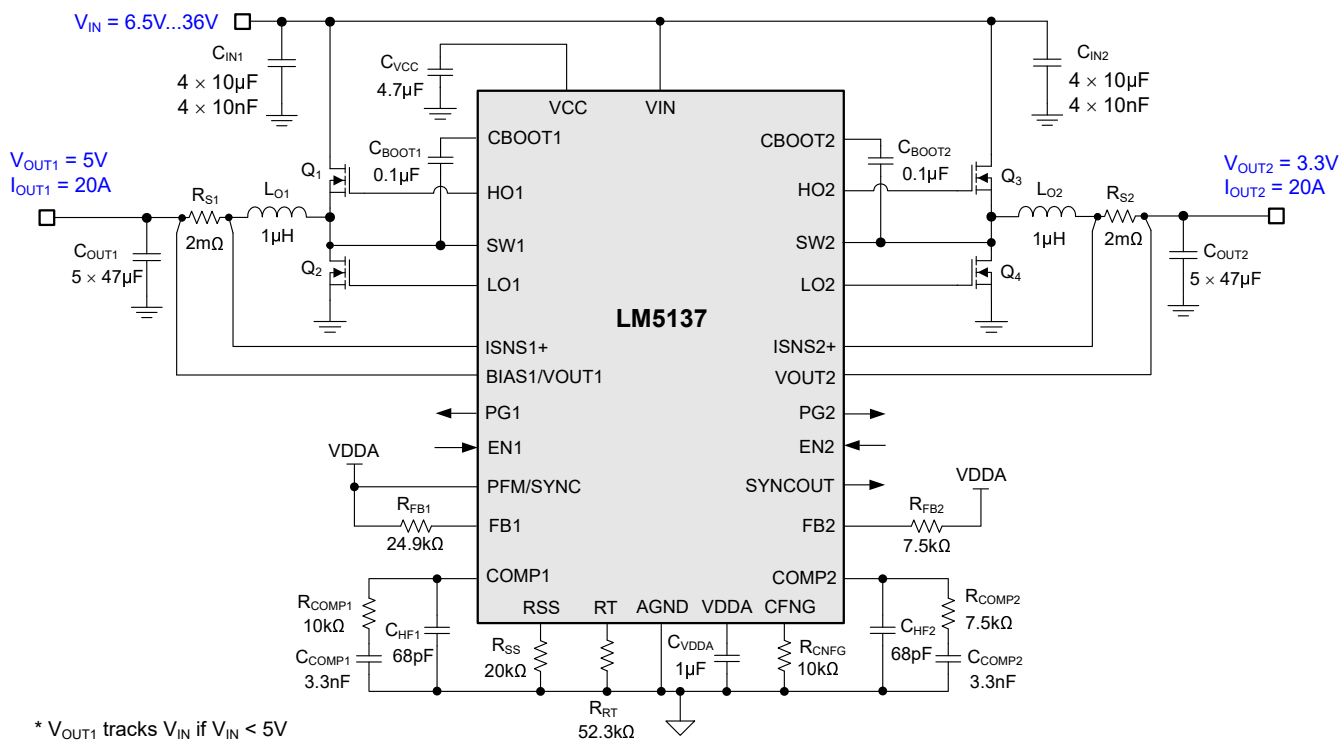
图 8-4. 采用 LM5137 降压稳压器且开关频率为 440kHz 时的应用电路 1
