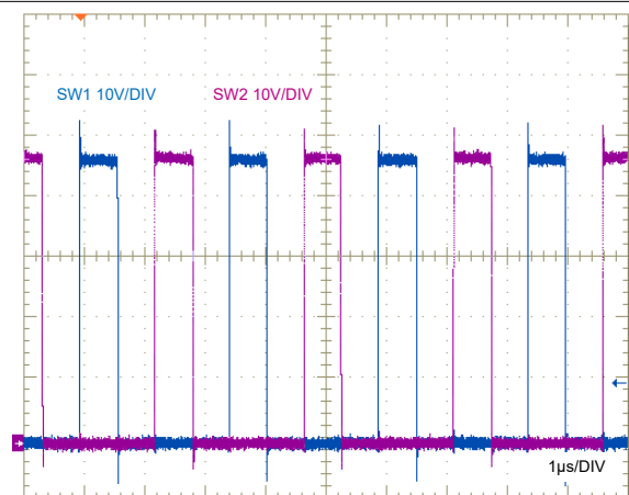
图 6-6. 开关节点电压
