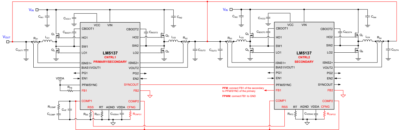
图 7-9. LM5137 配置为单输出交错式操作时的多相稳压器原理图
