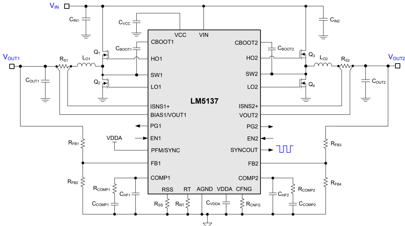
图 7-1. LM5137 双路输出稳压器原理图
