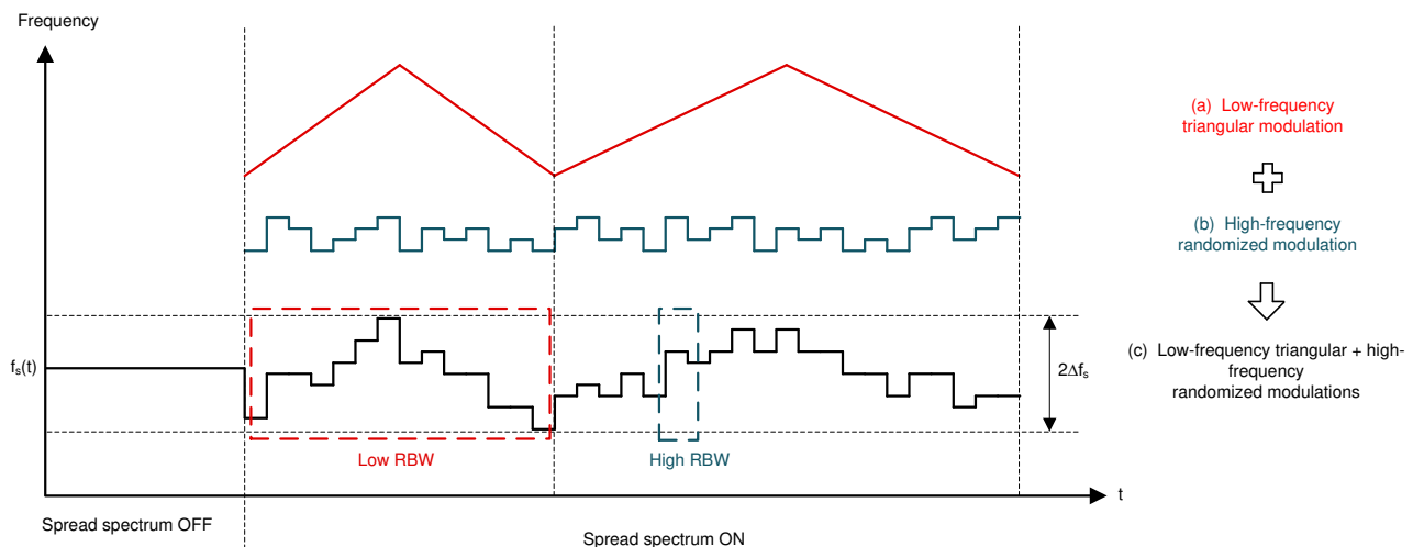
图 7-3. DRSS 实现
