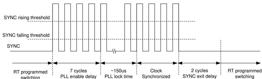
图 7-9. External Clock Synchronization
