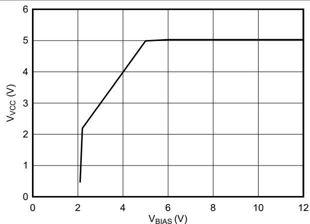
图 6-8. V_{BIAS} vs V_{VCC}
