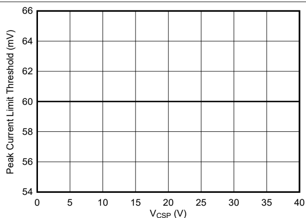
图 6-10. Peak current limit threshold V_{CLTH} vs V_{CSP}
