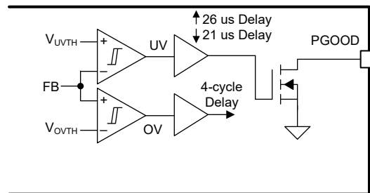
图 7-7. PGOOD Indicator
