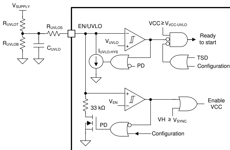
图 7-1. EN/UVLO Circuit
