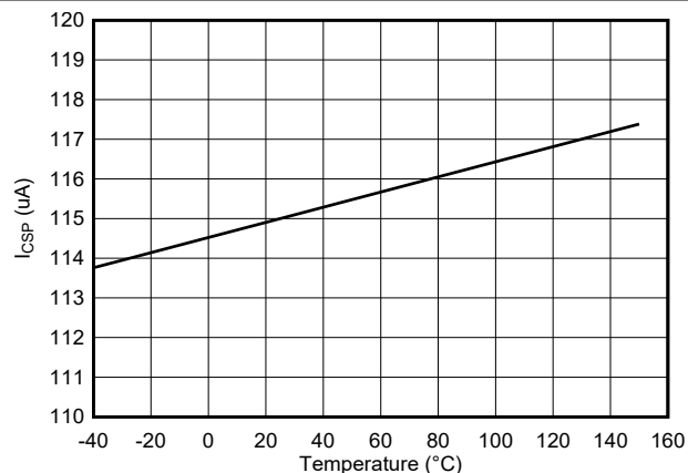
图 6-14. I_{CSP} vs temperature (active mode) V_{CSP} = 3\text{ V}
