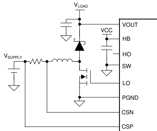
图 8-9. Non-synchronous boost configuration
