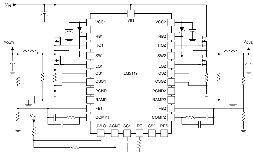
简化应用电路
