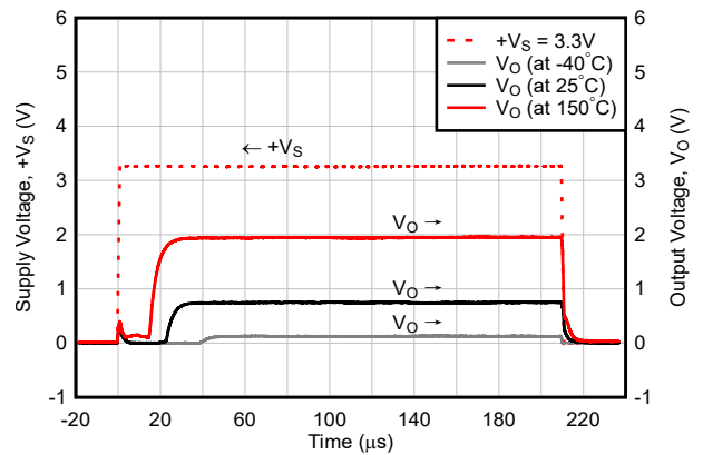
图 6-30. +V_S = 3.3\text{V} 阶跃时的启动响应 (当 t_r = 1\mu\text{s} 、无 C_{\text{Load}} 和 C_{\text{By-pass}} 时)
