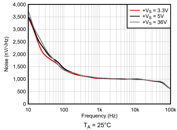
图 6-35. 输出噪声密度
