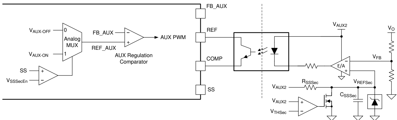
图 7-8. Soft-Start Function
