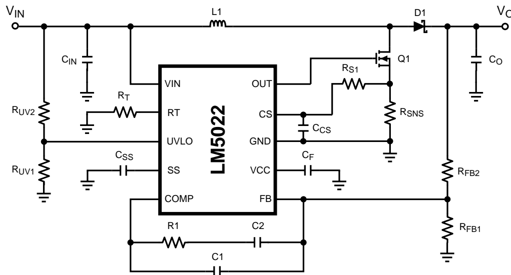
典型应用
