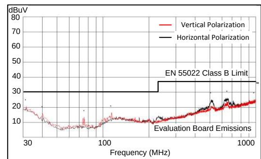
辐射发射图
