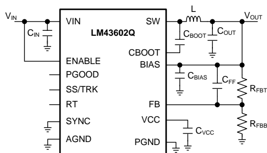
简化原理图
