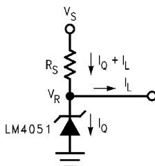
图 8-1. 并联稳压器
