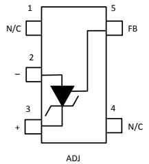
图 4-5. DCK 封装 5 引脚 SC70 顶视图
