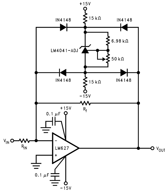
图 8-4. 有界放大器
