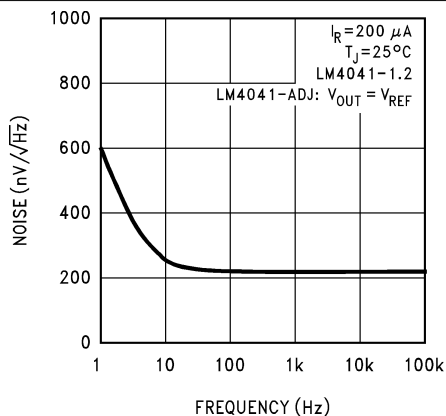
图 5-3. 噪声电压
