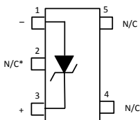
图 4-2. DCK 封装 5 引脚 SC70 顶视图
