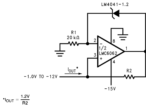
图 8-8. 精密 1 μA 至 1mA 电流吸收
