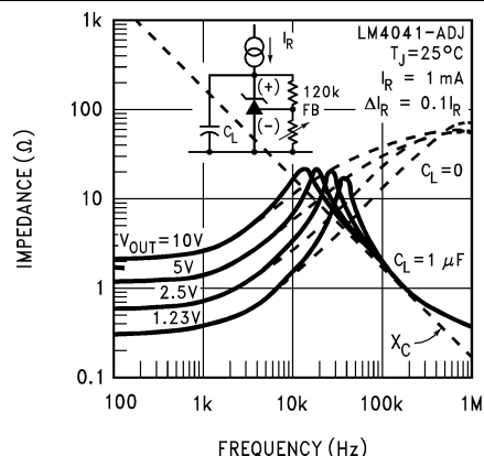
图 5-10. 输出阻抗与频率间的关系
