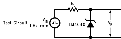
图 6-1. 测试电路
