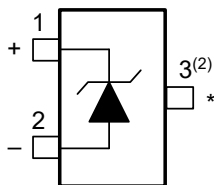
图 4-1. DBZ 封装 3 引脚 SOT-23 顶视图
