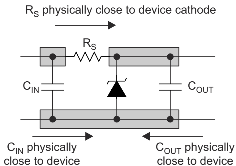
图 8-9. 布局图
