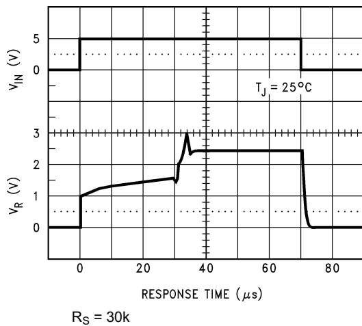
图 5-6. 输入电压阶跃响应 LM4040-N-2.5
