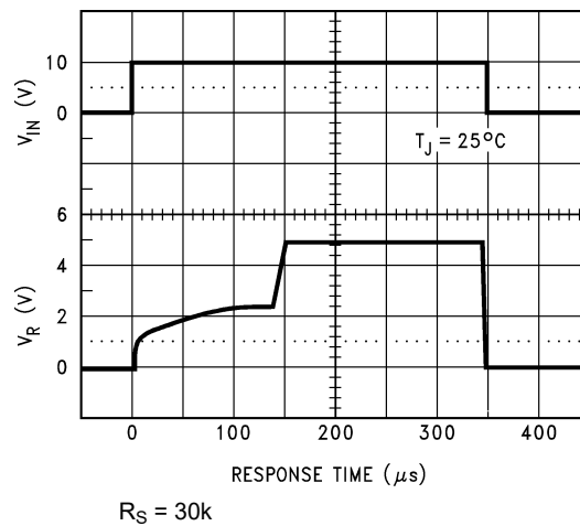
图 5-7. 输入电压阶跃响应 LM4040-N-5
