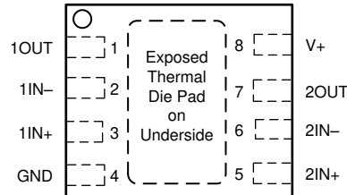
图 4-1. D、DGK、JG、P、PS、DDF 或 PW 封装 8 引脚 SOIC、VSSOP、PDIP、SO 或 TSSOP 顶视图
